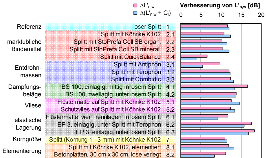
Bild 5: Einzahlangaben zu den in Bild 4 dargestellten Messkurven. Neben der Verbesserung des bewerteten Norm-Trittschallpegels durch die Schüttung, \Delta L'_{n,w} , ist außerdem die auf die Summe L'_{n,w} + C_i bezogene Verbesserung dargestellt (hierbei bezeichnet C_i den Spektrum-Anpassungswert für den Trittschallpegel nach DIN EN ISO 717-2).
