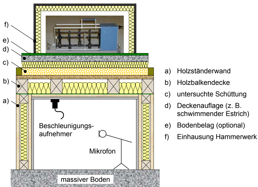
Bild 2: Messaufbau zur Untersuchung der akustischen Wirkung von gebundenen Schüttungen. Der Aufbau bestand aus dem Ausschnitt einer bauüblichen Holzbalkendecke (Maße L \times B = 1,5 \text{ m} \times 1,25 \text{ m} ), die auf vier Wänden in Holzständer-Bauweise auflag und unter der sich eine Messkammer mit einem Volumen von ca. 1,1 \text{ m}^3 befand.
