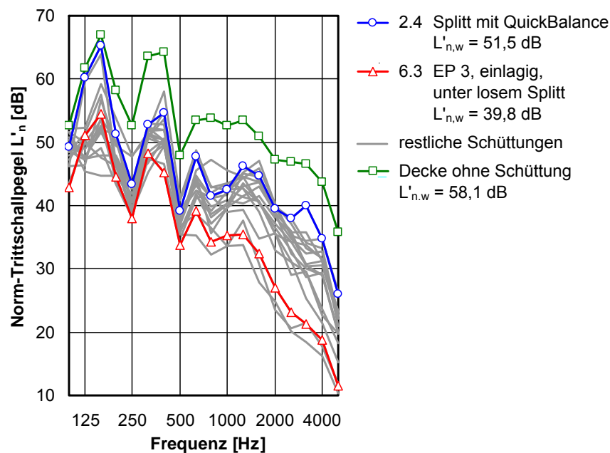
Bild 4: Norm-Trittschallpegel einer Holzbalkendecke bei Beschwerung mit achtzehn verschiedenen Schüttungen. Die Messungen erfolgten in Verbindung mit einem schwimmenden Estrich in mineralischer Bauweise. Die Schüttung mit dem höchsten Wert des bewerteten Norm-Trittschallpegels L'_{n,w} (also die akustisch ungünstigste Variante) ist als blaue Kurve, die Schüttung mit dem niedrigsten Wert als rote Kurve dargestellt. Die Messkurven für alle übrigen Schüttungen sind als graue Linien eingezeichnet. Zum Vergleich ist außerdem der Trittschallpegel für die Decke ohne Schüttung wiedergegeben (grüne Kurve).
