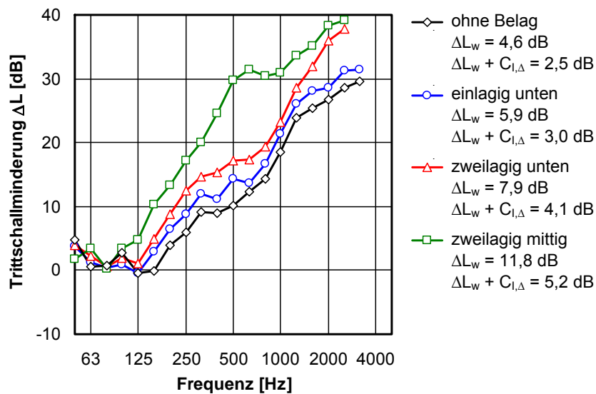
Bild 1: Verbesserung der Trittschallminderung eines Trockenestrichs durch Bedämpfung der Bodenplatte mittels aufgeklebter Bitumenbeläge. Bei der grünen Kurve waren die Beläge mittig in die Bodenplatte integriert (Sandwichbauweise).
