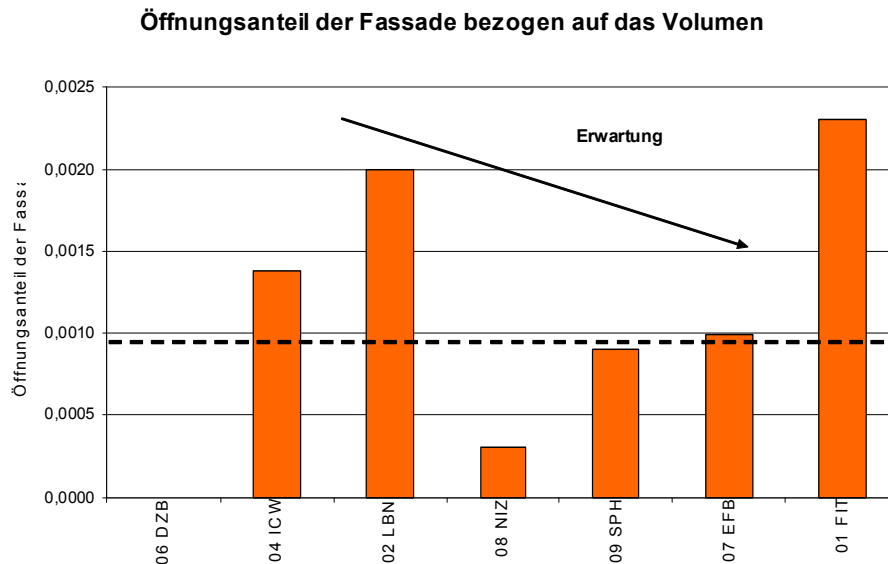
Abbildung 8 Öffnungsanteil der Außenfassaden in der Rangfolge der Überhitzung der Atrien
