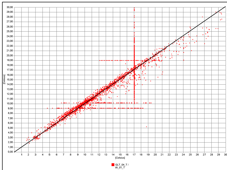
Abbildung 101 GLT-Außentempersensor und Außentempersensor der Wetterstation auf der Dachfläche , x-y-Abhängigkeit (GLT 04 GLT-Sensor auf y-Achse; W_01
