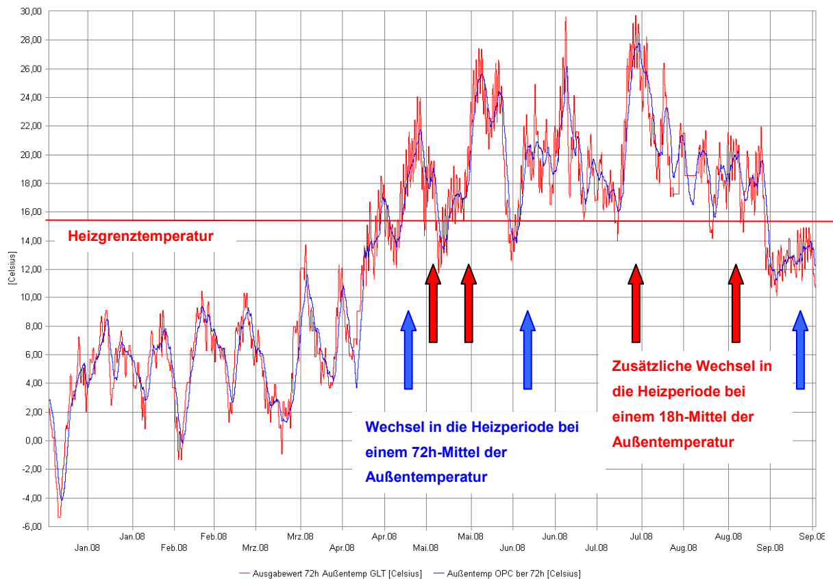
Abbildung 50 Gleitendes Mittel der Außentemperatur: Ausgabewert der GLT (18h-Mittel) und selber berechnetes 72h-Mittel
