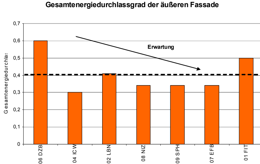
Abbildung 9 Gesamtenergiedurchlassgrad der Außenfassaden in der Rangfolge der Überhitzung der Atrien
