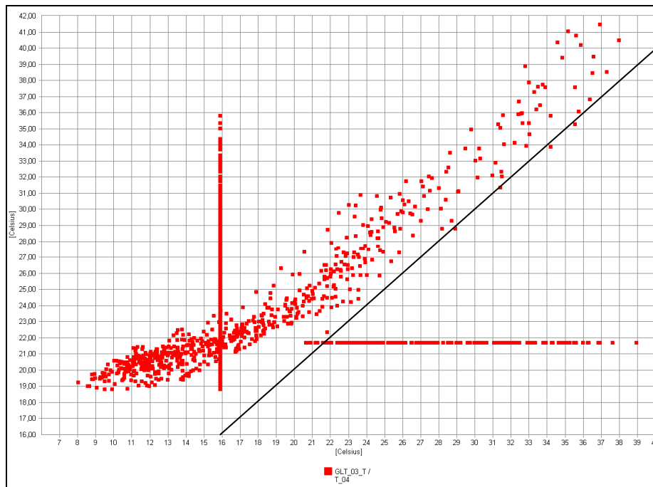
Abbildung 97 Abgleich oberer Temperatursensor mit eigenen Temperaturmessungen (GLT 03 GLT Sensor auf Y-Achse; T_04 IGS Sensor auf x-Achse)
