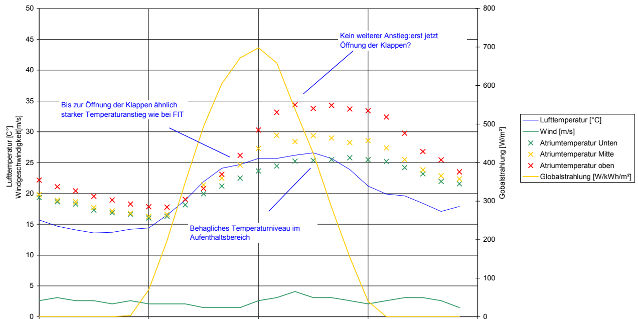
Abbildung 10 Tagesverlauf der Atrientemperaturen im Objekt und Außenklimabedingungen
