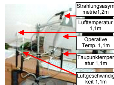
Mobile-LAB während einer Messung am Arbeitsplatz
