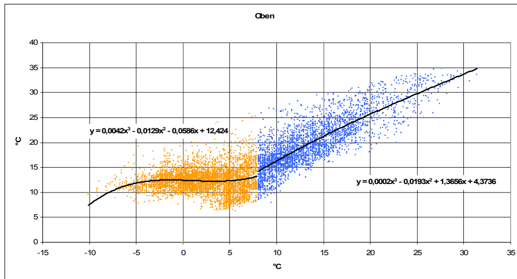
Abbildung 109 Approximierung der gemessenen Abhängigkeit der Atriumtemperatur von der Außentemperatur, oberster Ebene
