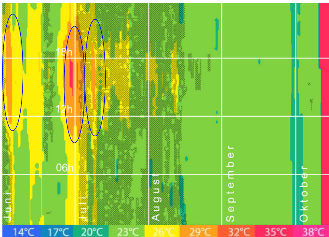
Abbildung 79 Carpetdiagramm mittlere Atriumtemperatur und Klappenöffnung für das NIZ
