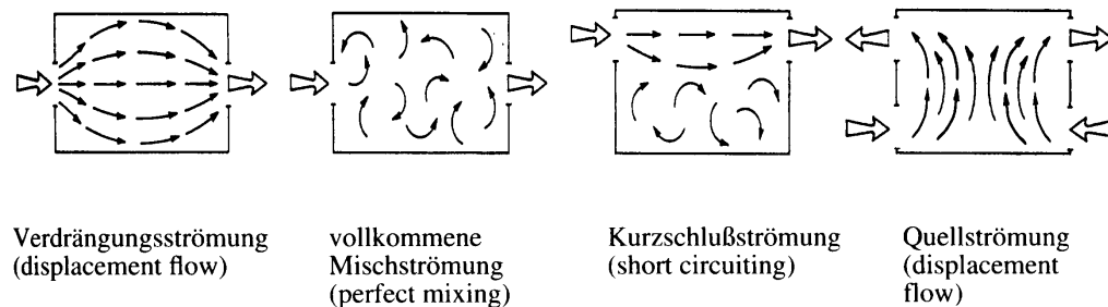
Abbildung 26 Grundformen der Raumströmung nach [Recknagel]
