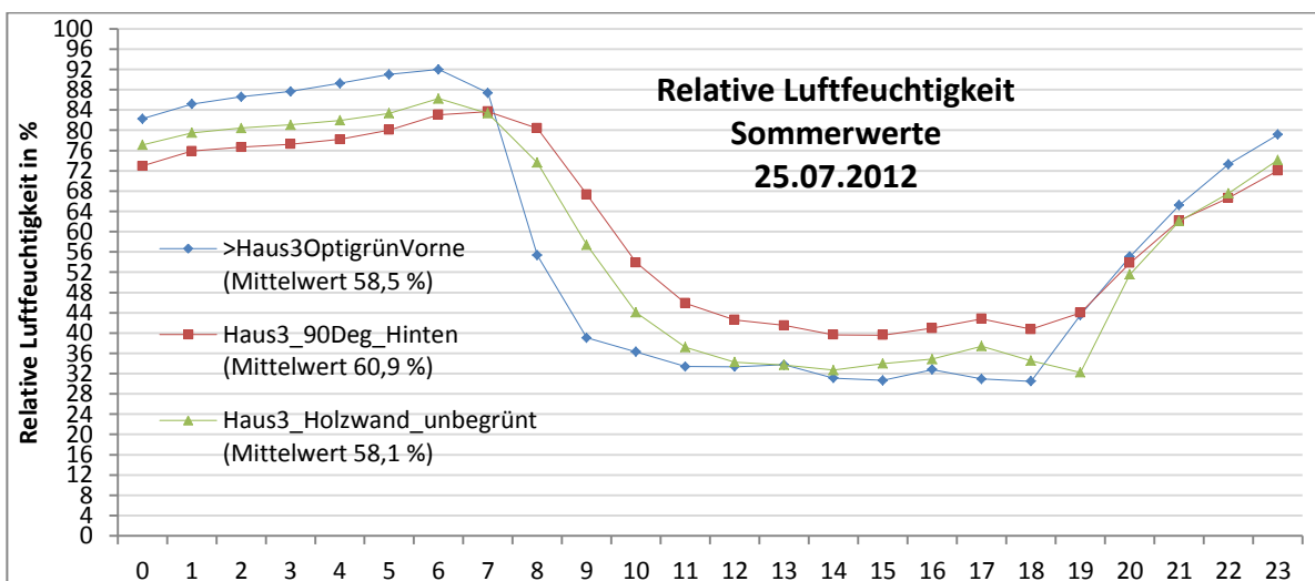
Abb. 2.12: Exemplarischen Tageswerte der relativen Luftfeuchtigkeit, Beispiel des Tagesgang eines Sommertages vom 25.07.2012, vor- und hinter einer begrünten Wand, sowie vor einer unbegrünten Holzwand.
