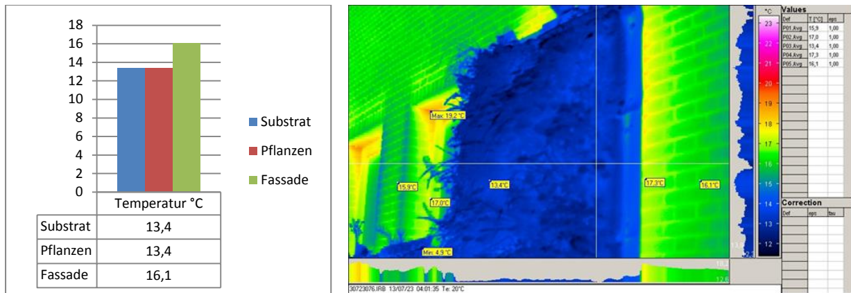
Abb. 2.48: Infrarot-Nachtfoto mit “Infratec-Varioscan” Kamera, WB Sempergreen Südfassade.
