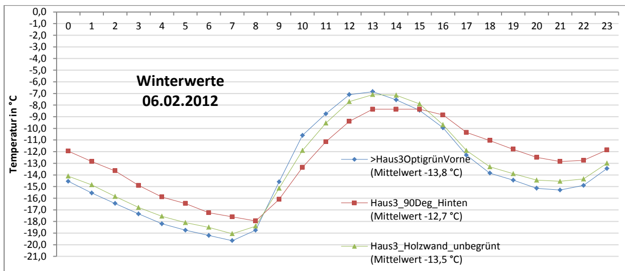
Abb. 2.13: Exemplarischen Tageswerte eines kalten Wintertages, 06.02.2012: Temperaturen, vor- und hinter einer begrünten Wand, sowie vor einer unbegrünten Holzwand.
