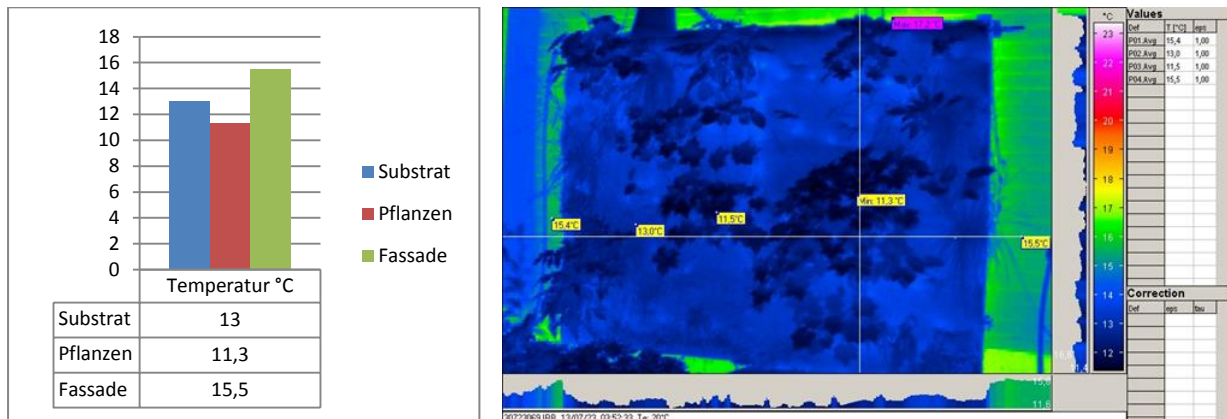
Abb. 2.50: Infrarot-Nachtfoto mit “Infratec-Varioscan” Kamera, Geovlies WB (Vertiko).
