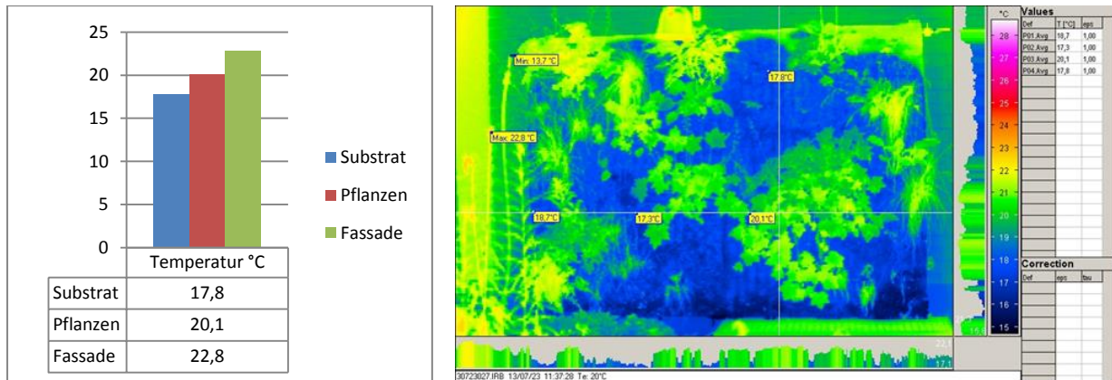
Abb. 2.49: Infrarot-Tagesfoto mit “Infratec-Varioscan” Kamera, Geovlies WB (Vertiko).
