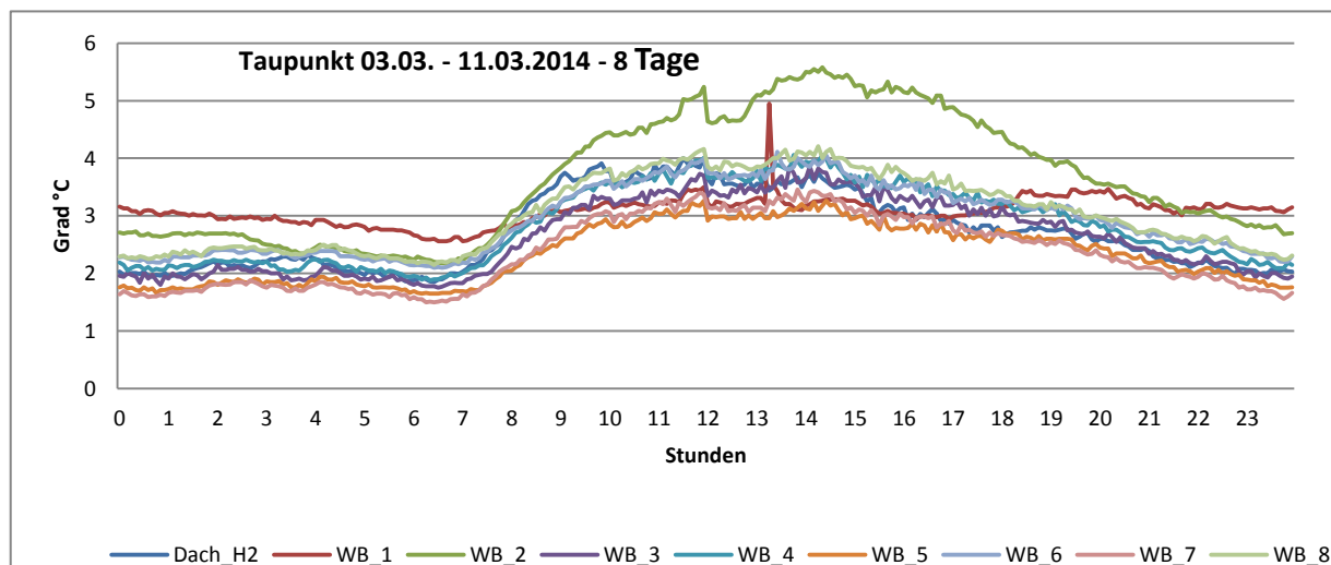
Abb.2.30: Taupunkt 03.03.2014 – 11.03.2014, für 8 Tage.
