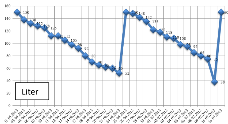
Abb. 2.7: Täglicher Wasserverbrauch der begrünten Innenwand Mai-Juli 2013 (Angabe in Liter Wassermenge im Vorratsbehälter).
