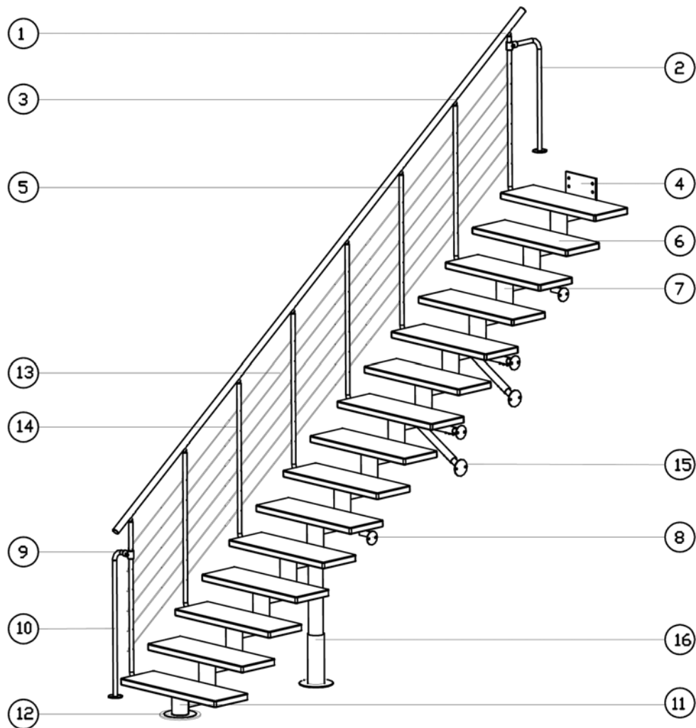
Elementy schodów modułowych ATRIUM SEGMENT
