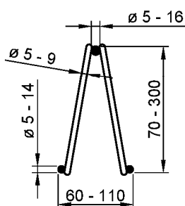
Bild 2: E-Gitterträger
