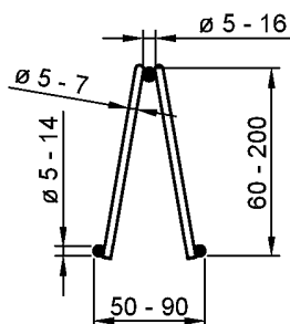
Bild 1: D-Gitterträger
