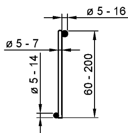
Bild 3: DH-Gitterträger
