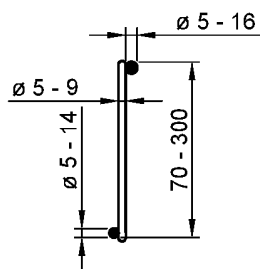
Bild 4: EH-Gitterträger
