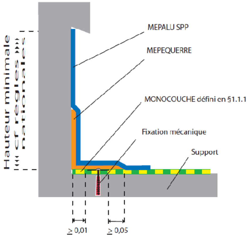
FIGURE 1 : Relevé d'un système monocouche fixé mécaniquement
