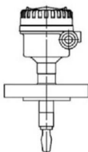
Flanschmontage (Standardlänge)
