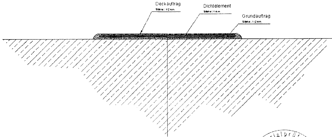
Abbildung 1: Aufbau des Tricoflex Abklebesystem über einer Arbeitsfuge
