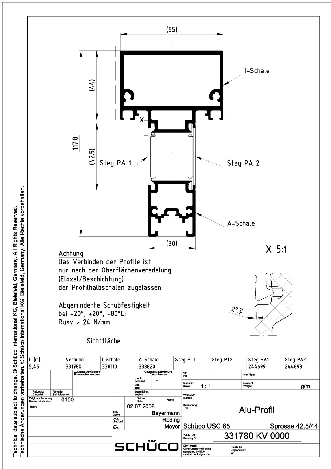
Bild 1 geprüftes Profil
