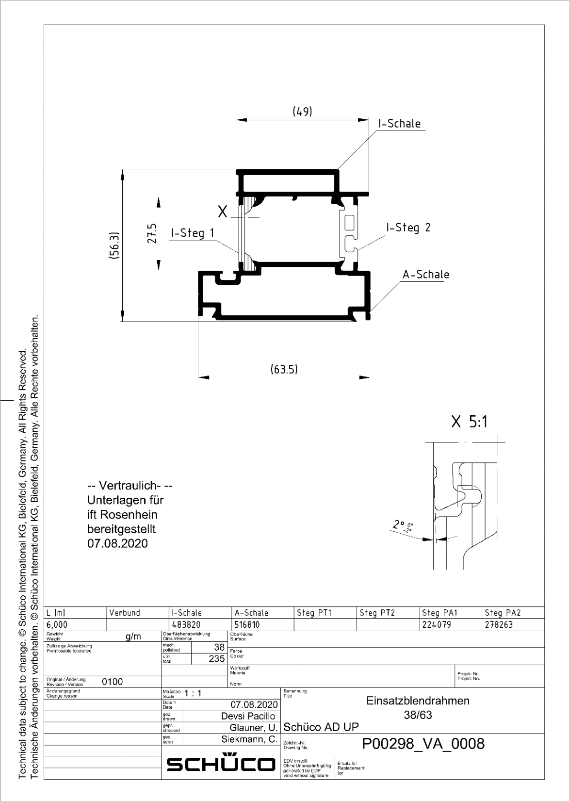
Bild 1 geprüftes Profil
