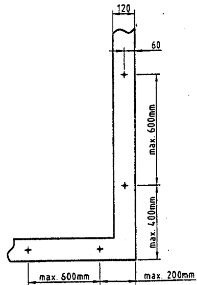
Dübelbefestigung des Rahmens
