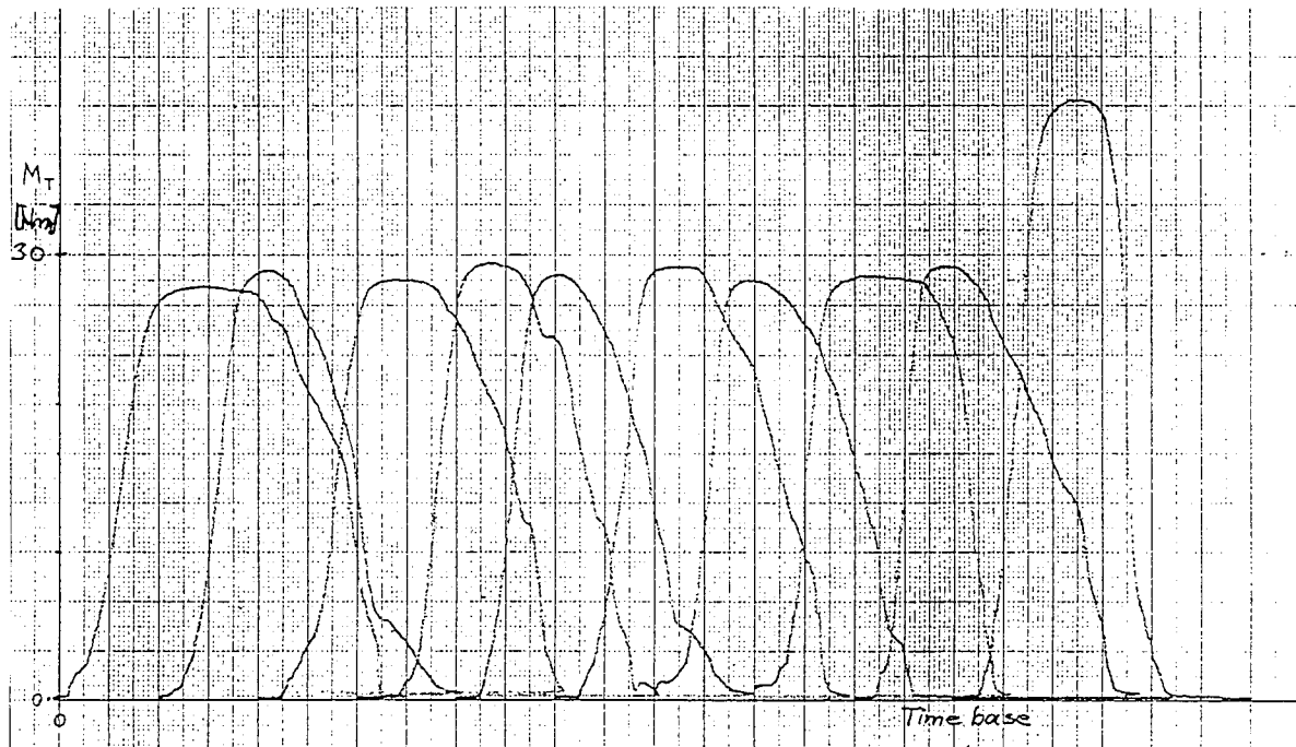
Bild 14: Holzschraube 10 x 100
