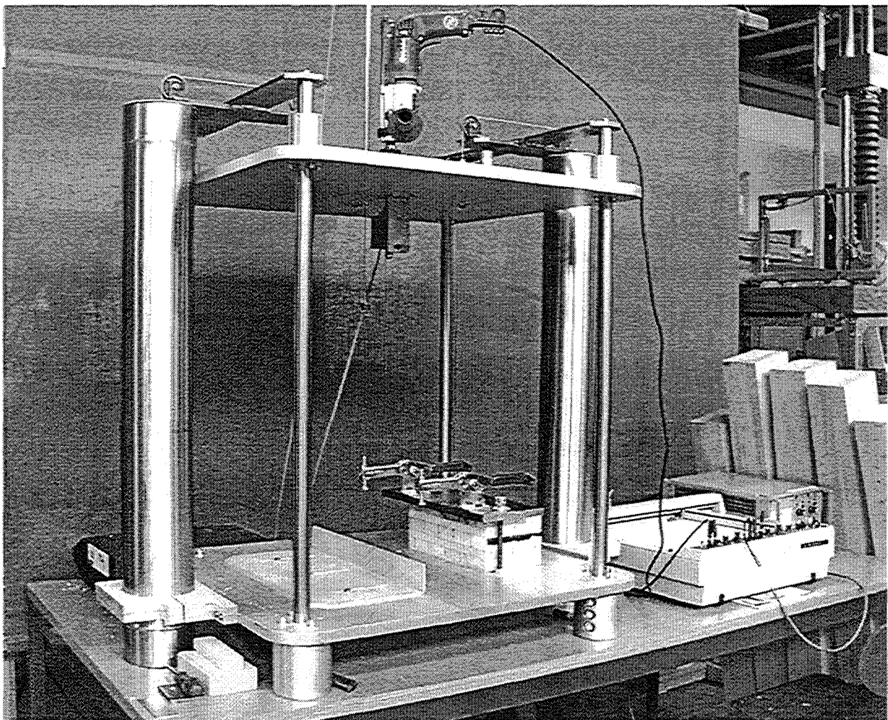
Bild 2: Drehmoment-Meßvorrichtung
