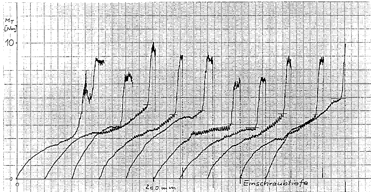
Bild 6: Würth - Schraube 6 x 120 in Fichte, tangential
