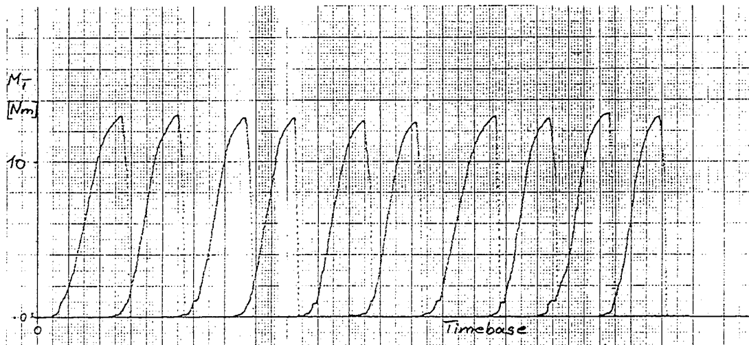
Bild 12: SFS - Schraube 6,5 x 130
