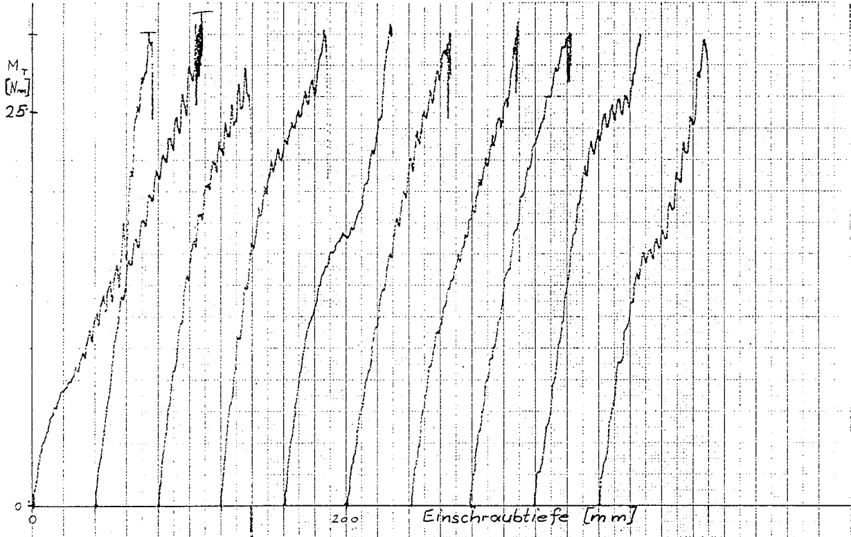
Bild 9: Holzschraube 10 x 100 in Buche, radial
