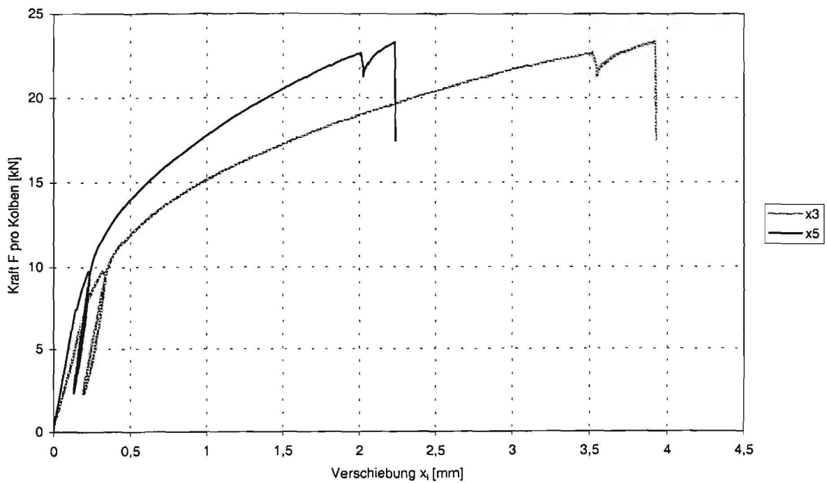
Abbildung C-14: Last-Verformungsverformungsdiagramm der Verschiebung x_3 und x_5 zwischen Holz und Beton des Trägers NAG-1
