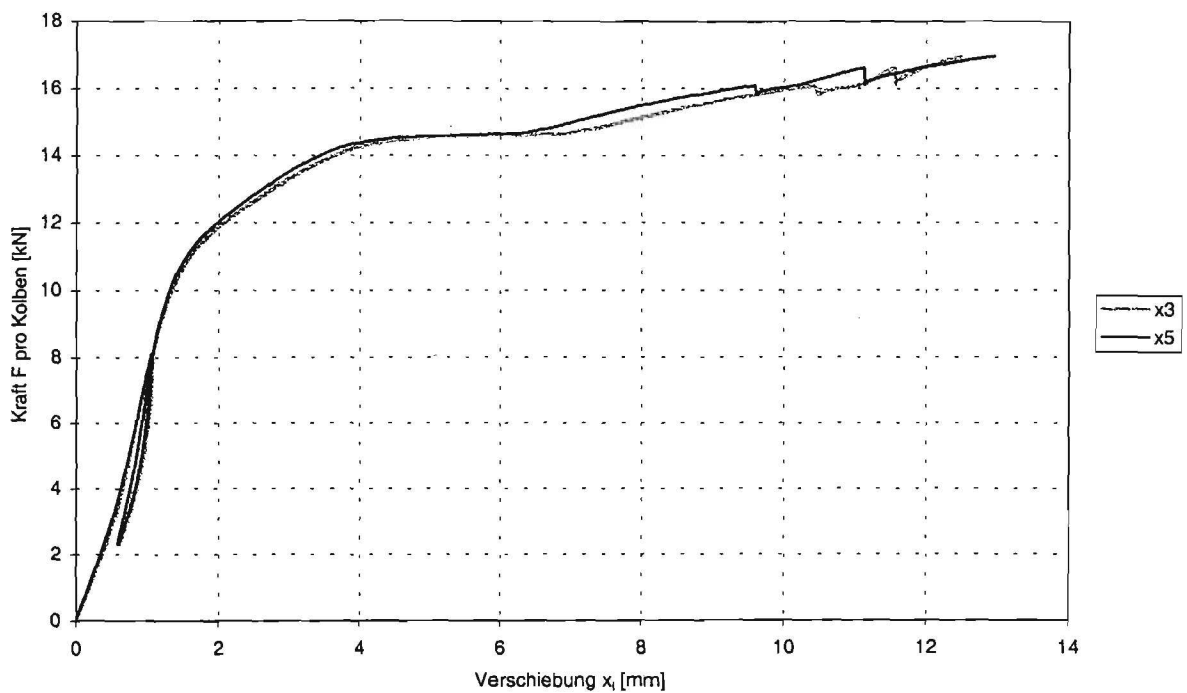
Abbildung C-10: Last-Verformungsverformungsdiagramm der Verschiebung x_3 und x_5 zwischen Holz und Beton des Trägers SCH-2
