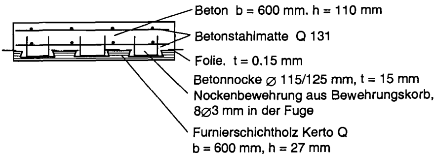
Abbildung A-3: Querschnitte der Holz-Beton-Verbundträger mit unterschiedlichen Verbindungsarten
