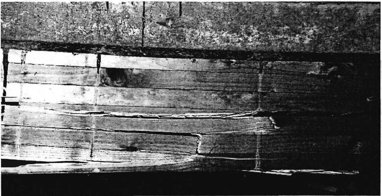
Abbildung C-8: Geprüfter Träger SCH-1
