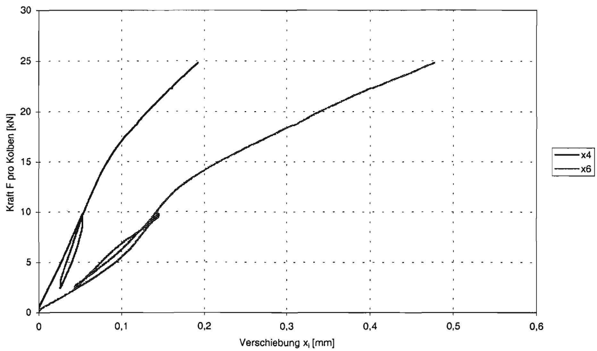
Abbildung C-31: Last-Verformungsverformungsdiagramm der Verschiebung x_4 und x_6 zwischen Holz und Beton des Trägers NPL-1
