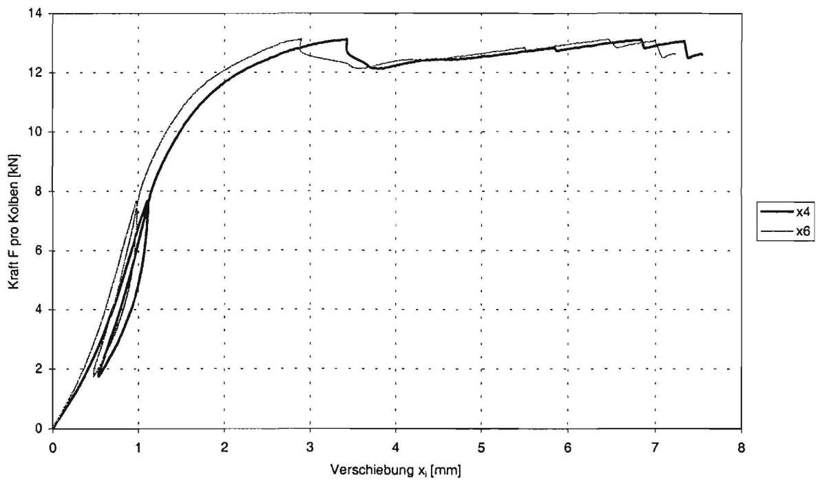
Abbildung C-7: Last-Verformungsverformungsdiagramm der Verschiebung x_4 und x_6 zwischen Holz und Beton des Trägers SCH-1
