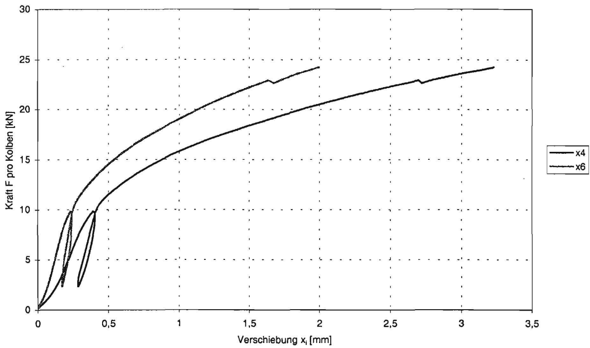
Abbildung C-19: Last-Verformungsverformungsdiagramm der Verschiebung x_4 und x_6 zwischen Holz und Beton des Trägers NAG-2
