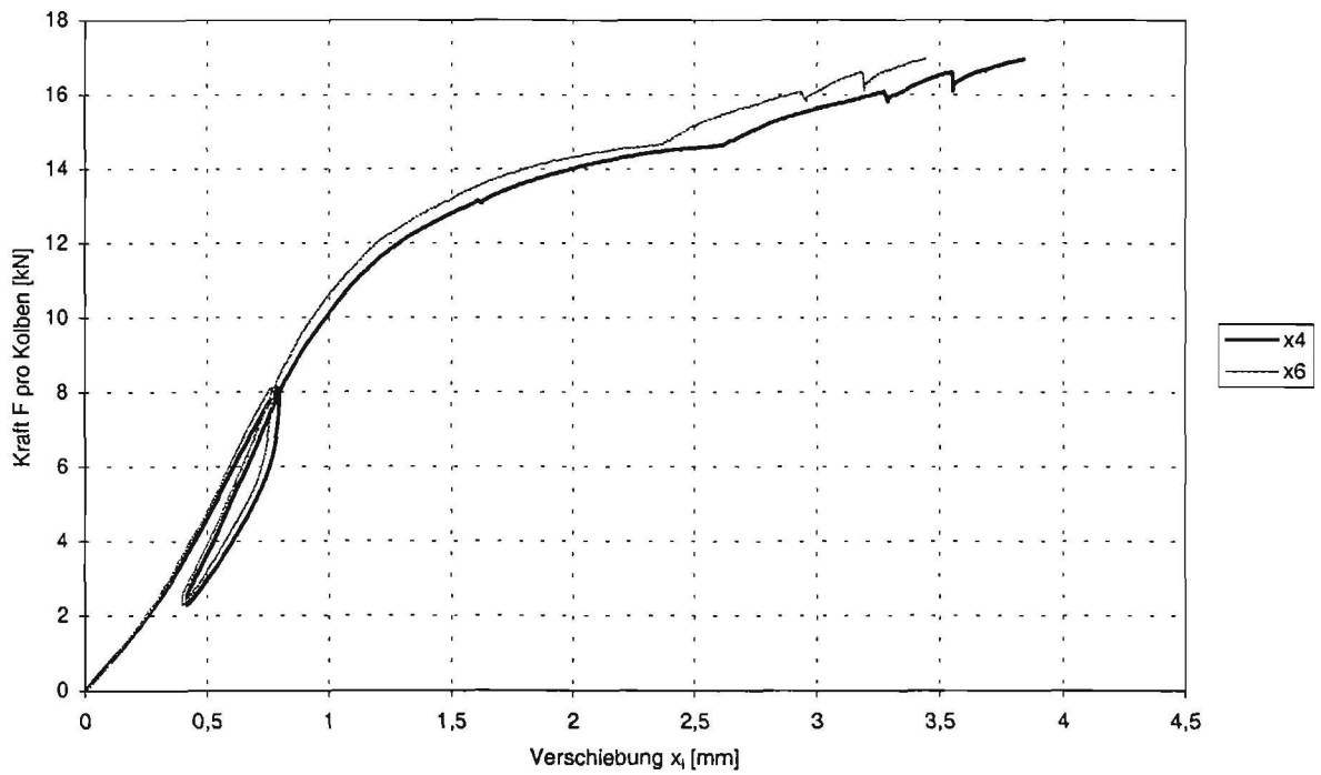
Abbildung C-11: Last-Verformungsverformungsdiagramm der Verschiebung x_4 und x_6 zwischen Holz und Beton des Trägers SCH-2
