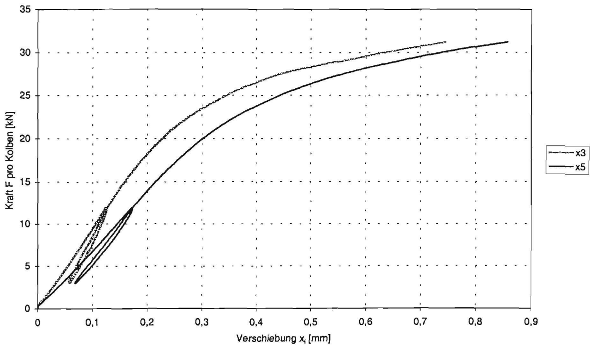
Abbildung C-22: Last-Verformungsverformungsdiagramm der Verschiebung x_3 und x_5 zwischen Holz und Beton des Trägers N+S-1
