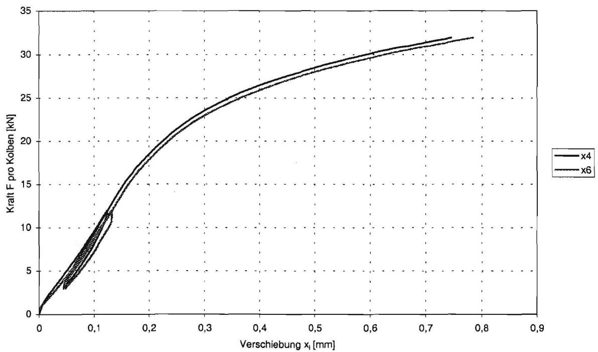
Abbildung C-27: Last-Verformungsverformungsdiagramm der Verschiebung x_4 und x_6 zwischen Holz und Beton des Trägers N+S-2
