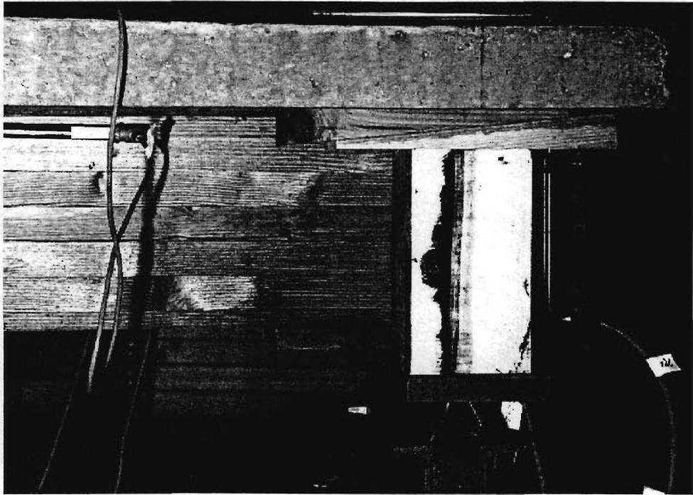
Abbildung C-3: Versuchsaufbau der Biegeversuche im Auflagerbereich (seitliche Abstützung)
