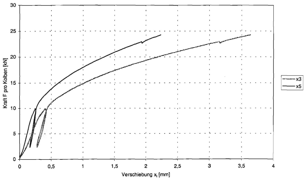
Abbildung C-18: Last-Verformungsverformungsdiagramm der Verschiebung x_3 und x_5 zwischen Holz und Beton des Trägers NAG-2
