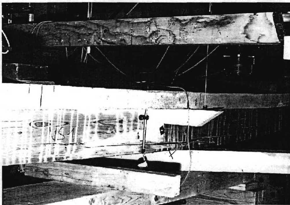
Abbildung C-24: Geprüfter Träger N+S-1
