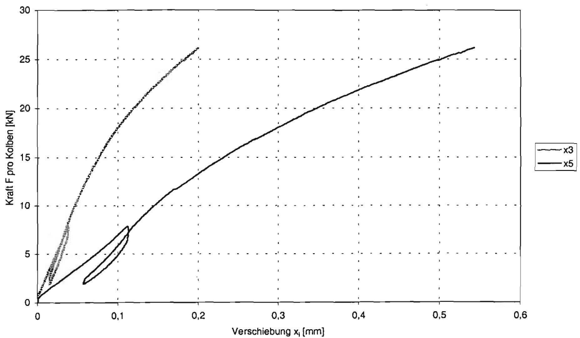
Abbildung C-34: Last-Verformungsverformungsdiagramm der Verschiebung x_3 und x_5 zwischen Holz und Beton des Trägers NPL-2
