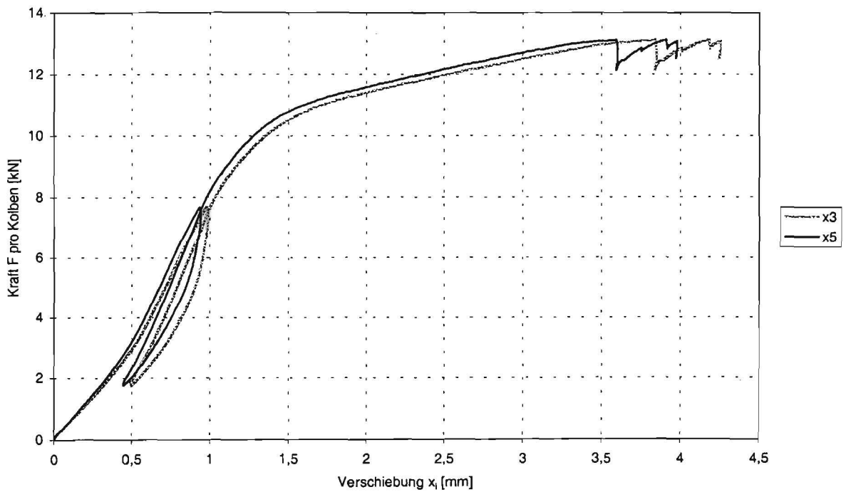
Abbildung C-6: Last-Verformungsverformungsdiagramm der Verschiebung x_3 und x_5 zwischen Holz und Beton des Trägers SCH-1
