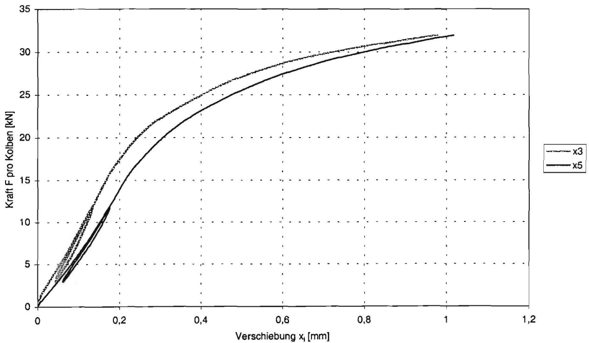
Abbildung C-26: Last-Verformungsverformungsdiagramm der Verschiebung x_3 und x_5 zwischen Holz und Beton des Trägers N+S-2
