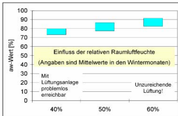
Abb. Änderung des aw-Wertes einer innen gedämmten Wand in Abhängigkeit von der relativen Raumlufffeuchtigkeit am Beispiel von 80 mm EPS Innendämmung ohne Dampfbremse [PHI 2006]
