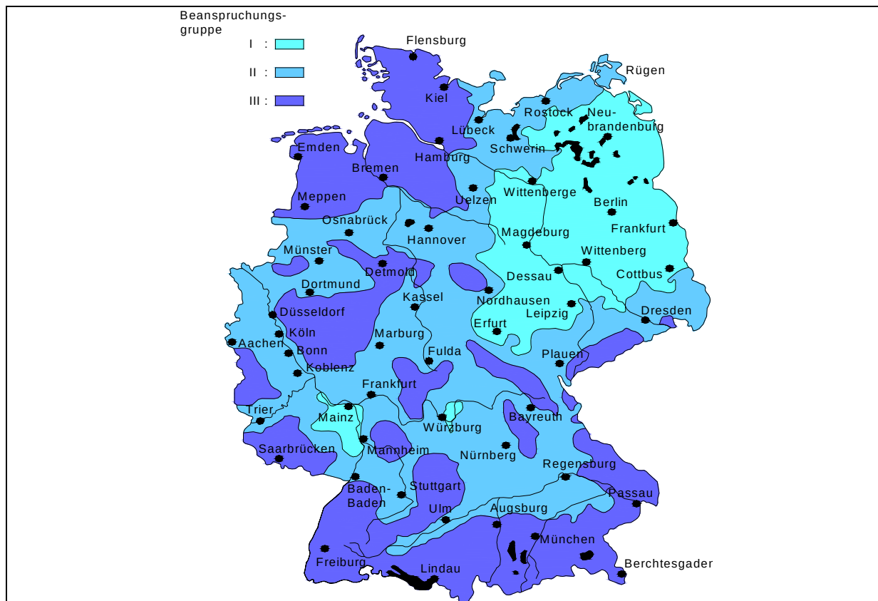
Abb. 2.4 Darstellung der regionalen Verteilung der Schlagregenbeanspruchungsgruppen in der Bundesrepublik Deutschland nach DIN 4108-3, Anhang C [DIN 4108-3]
