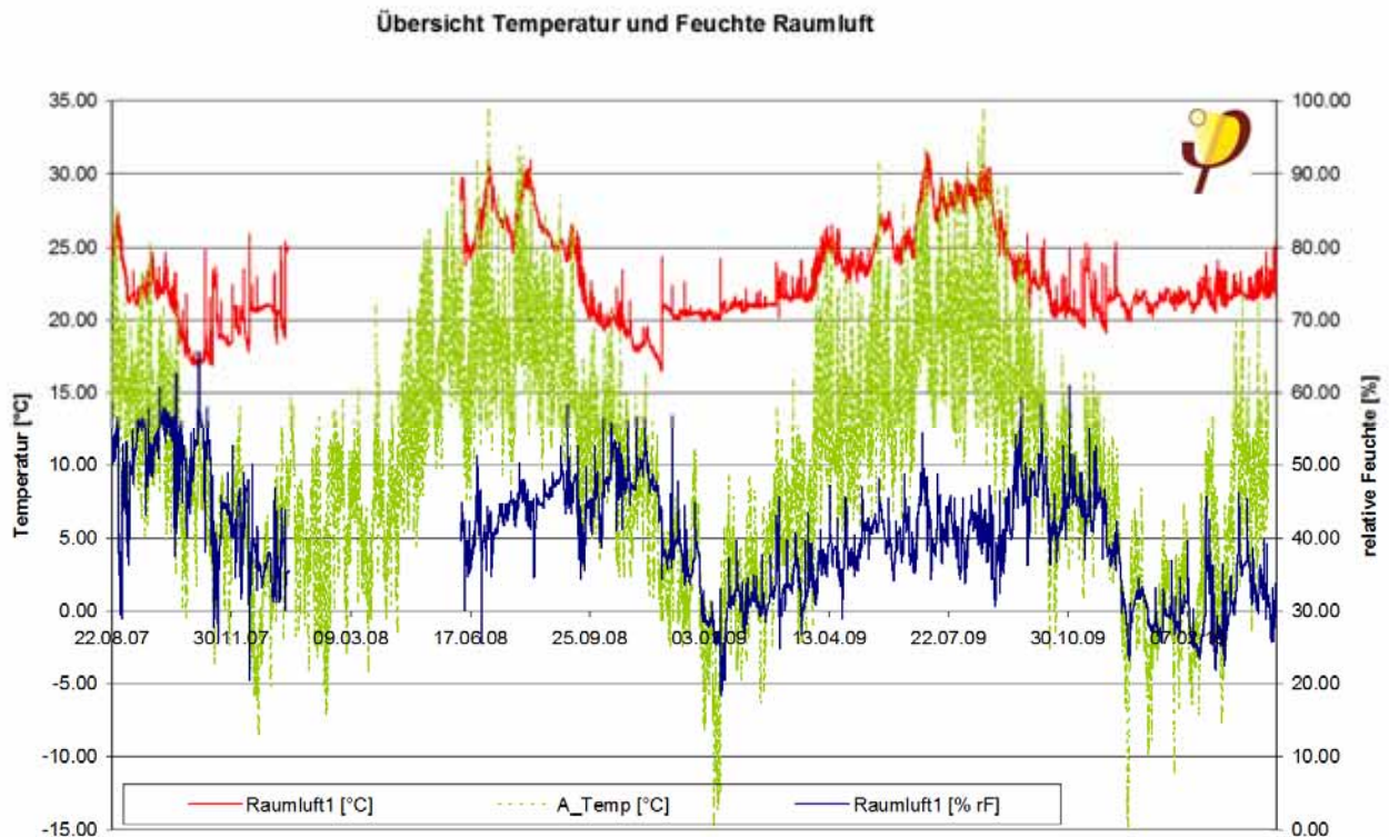
Abbildung 13. Stundenwerte von Temperatur und Feuchte der Innenraumluft, Außenlufttemperatur
