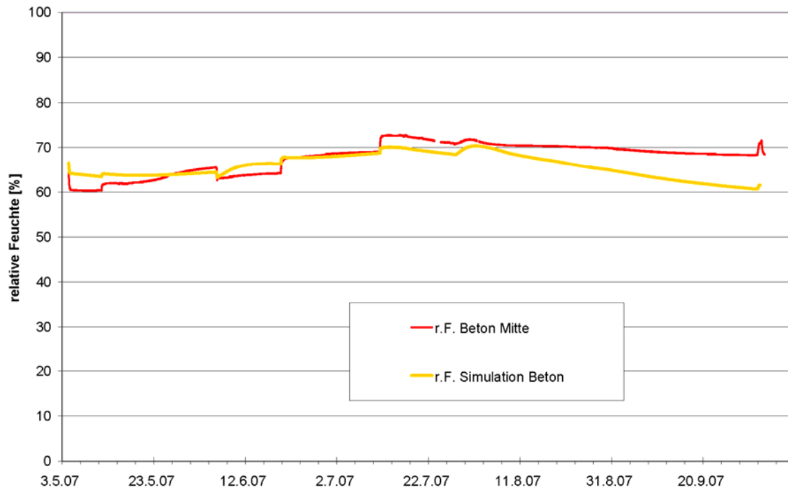
Abbildung 33: Vergleich der gemessenen und berechneten Verläufe der relativen Feuchte (Aw-Wert) im Beton
