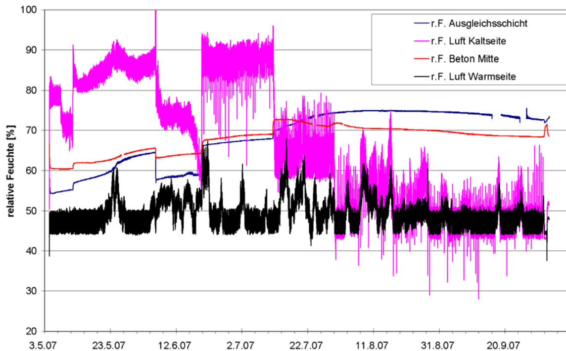
Abbildung 29: Relative Feuchte in Klimakammer und Probenkörper
