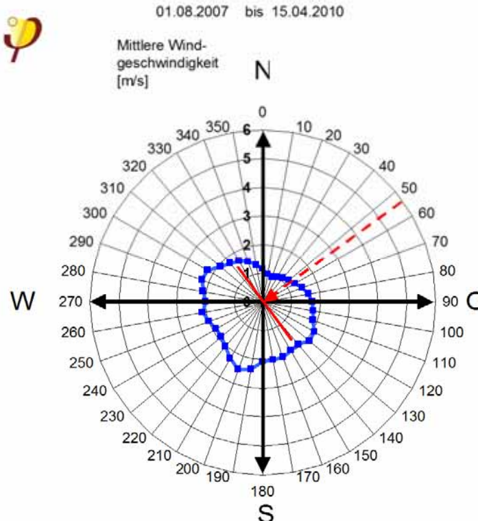
Abbildung 10.: Polardiagramm der Windverhältnisse im Gesamtzeitraum der Untersuchung, rot die Ausrichtung der innen gedämmten Gebäudewand mit Azimut-Pfeil
