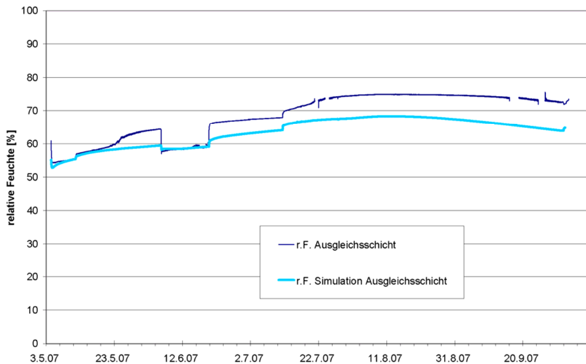
Abbildung 34: Vergleich der gemessenen und berechneten Verläufe der relativen Feuchte (Aw-Wert) in der Ausgleichsschicht
