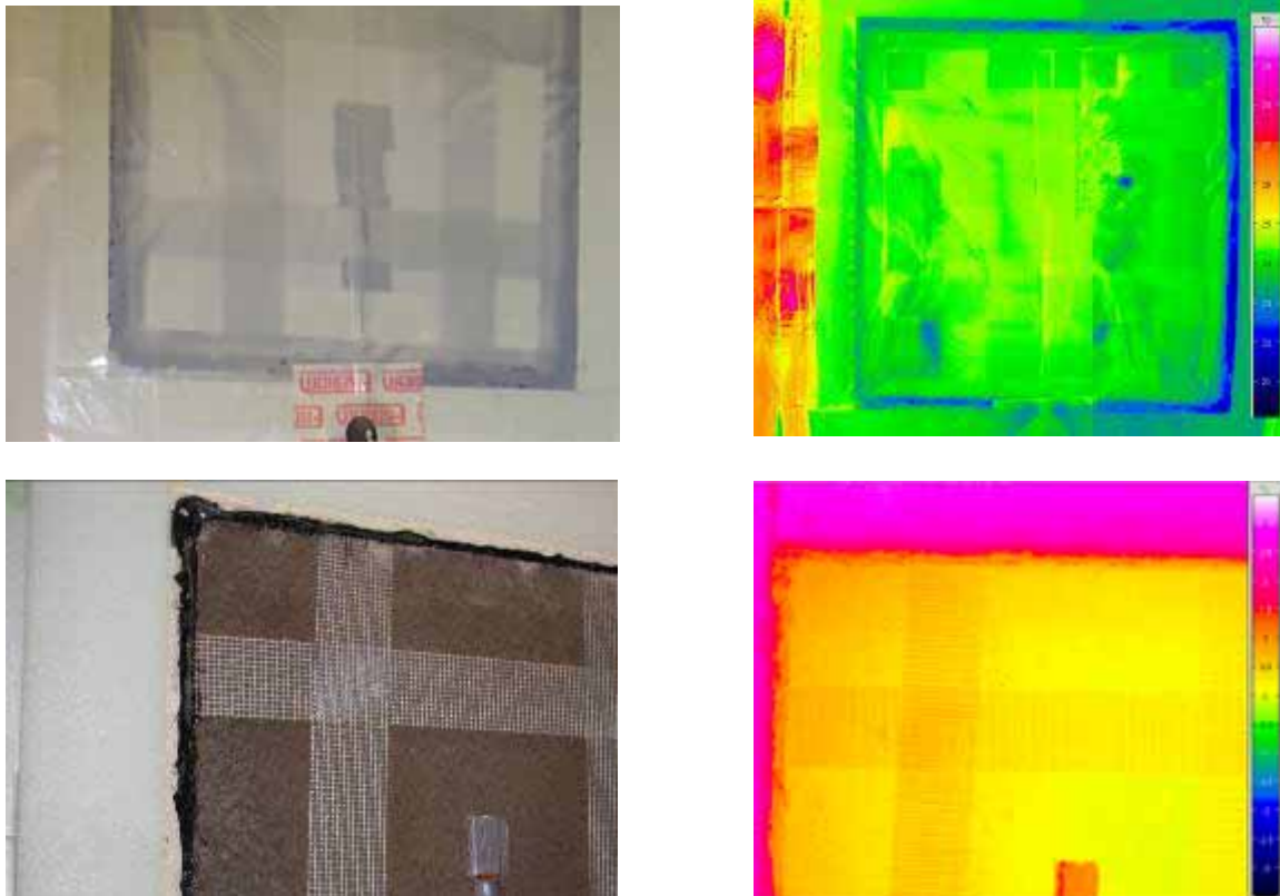
Abbildung 27: Fotos (links) und Infrarotthermografie (rechts) der Probe warmseitig (oben) bzw. kaltseitig (unten). Auf beiden Thermografien ist deutlich der Randeinfluss zu erkennen.
