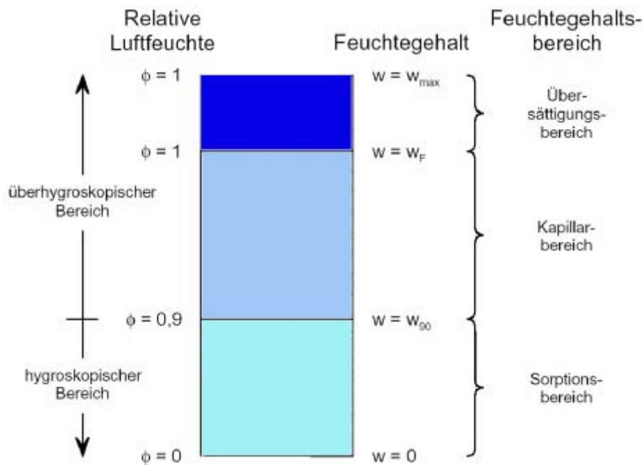
Abbildung 2: Feuchtegehaltsbereiche hygroskopischer Stoffe
