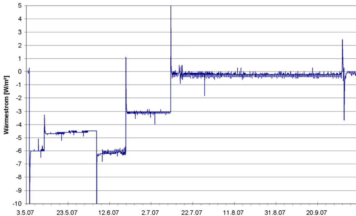
Abbildung 30: Wärmefluss auf dem VIP-Element (zwischen Ausgleichsschicht und VIP)
