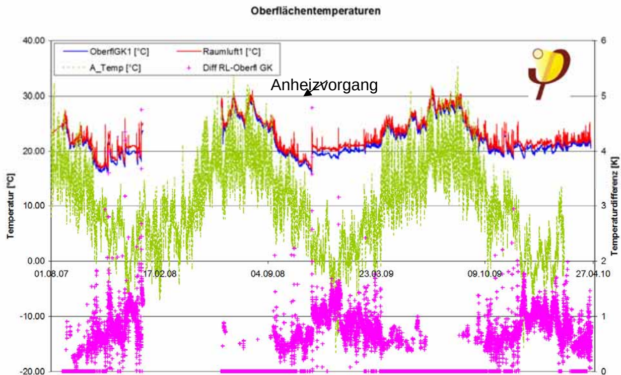
Abbildung 14. Stundenwerte der gemessenen Oberflächentemperatur der GK-Vorsatzschale, der Raumlufthtemperatur und Außenlufttemperatur im Vergleich mit den Temperaturdifferenzen der Raumlufth zu der GK-Oberfläch (magentafarben)
