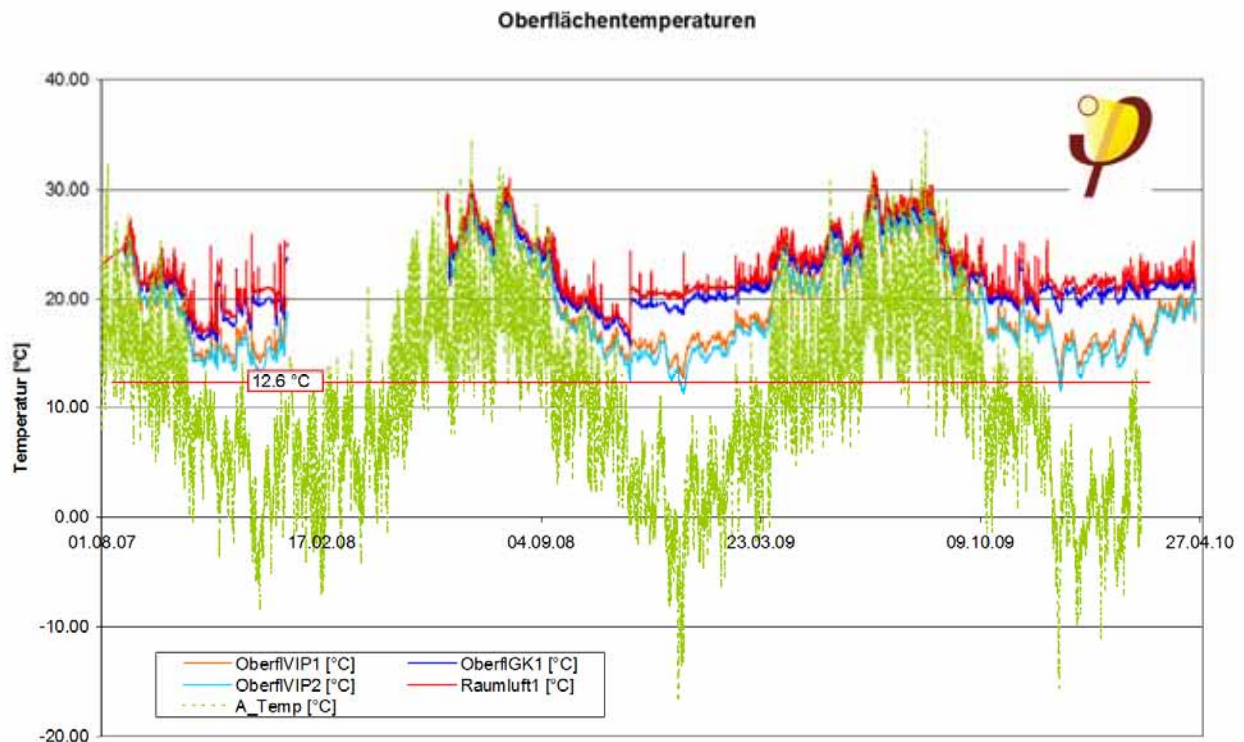
Abbildung 15. Stundenwerte gemessener Oberflächentemperaturen, der Raumlufttemperatur und Außenlufttemperatur
