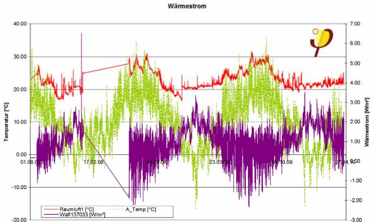
Abbildung 22. Gemessener Wärmestrom in der Regelfläche des Bauteilaufbaus (violett), Innentemperatur (rot) und Außentemperatur (grün)
