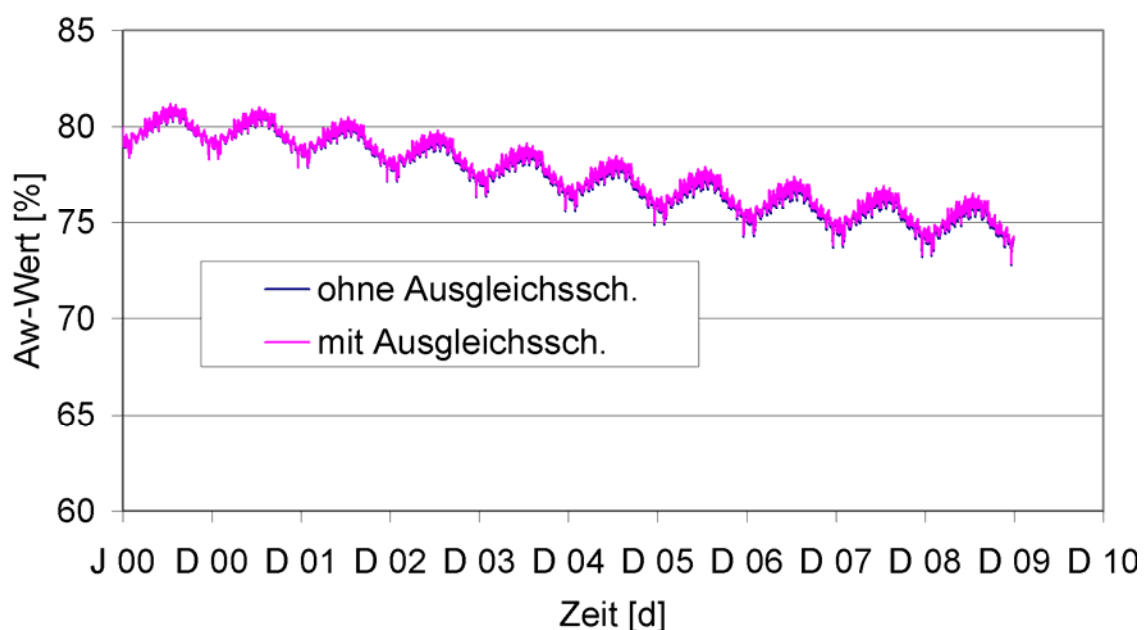
Abbildung 17. Verlauf der Wasseraktivität des Wandaufbaus mit Anstrich und Spachtelung jeweils mit und ohne Ausgleichsschicht zwischen Beton und VIP-Innendämmung; Simulationsergebnisse aus [Pfluger 2008]
