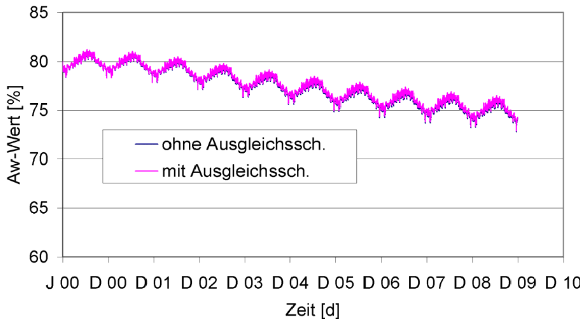
Abbildung 12: Verlauf der Wasseraktivität des Wandaufbaus mit Anstrich und Spachtelung jeweils mit und ohne Ausgleichsschicht zwischen Beton und VIP-Innendämmung
