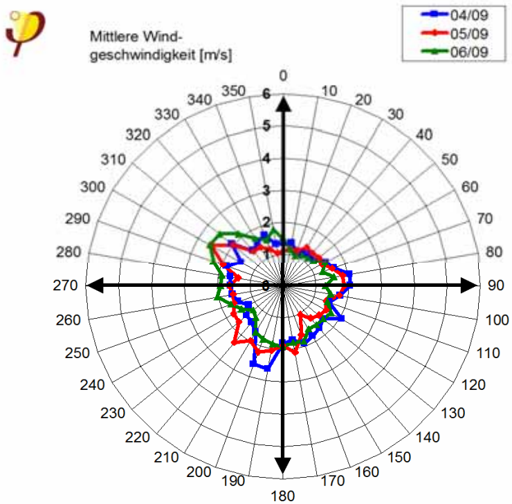
Anhang A 8: Polardiagramm Wind 2. Quartal 2009
