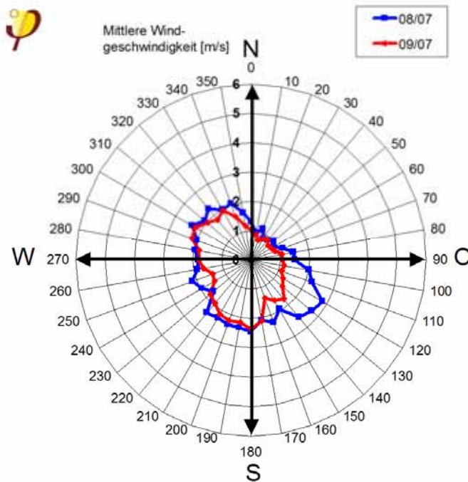
Anhang A 1: Polardiagramm Wind Aug-Sep 2007
