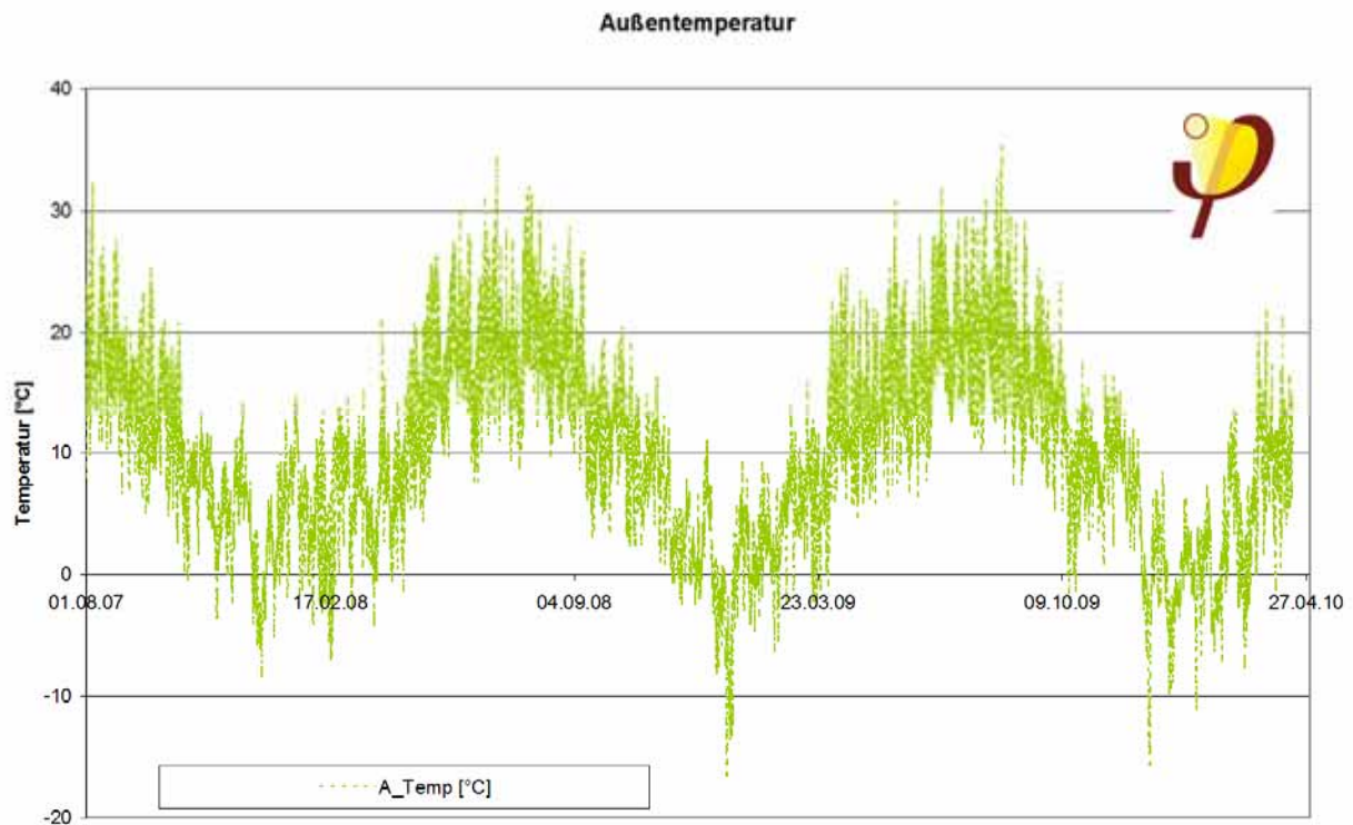
Abbildung 11. Stundenwerte der Außenlufttemperatur im Auswertezeitraum, Quelle [ZIMEN]
