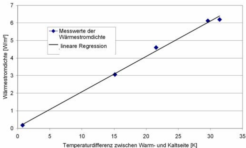
Abbildung 31: Messwerte und Regression der Wärmestromdichte in Abhängigkeit der Temperaturdifferenz
