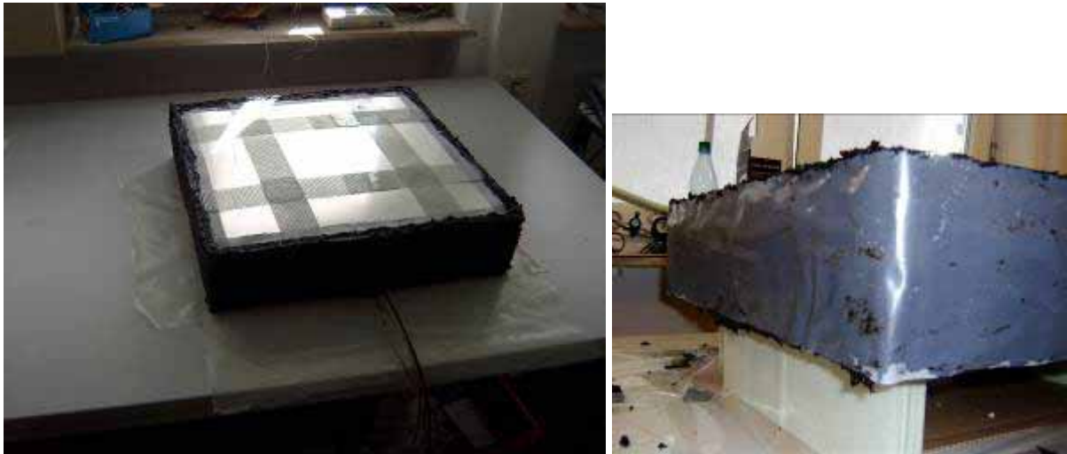
Abbildung 17 Randverbund aus Bitumendickbeschichtung und Sicherung durch Glasfaserbänder (links), Folie als Dampfsperre im Randverbundbereich (rechts)
