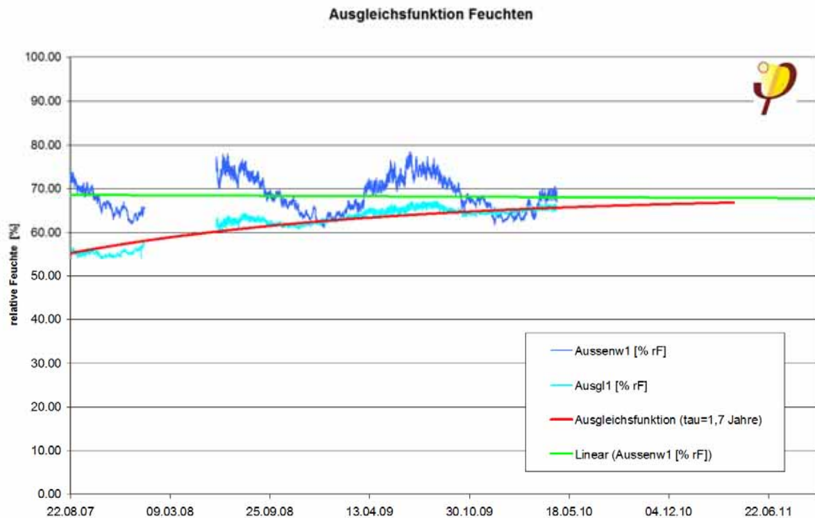
Abbildung 21. Mathematische Analyse des Feuchteausgleichsvorganges. Feuchteentwicklung in der Ausgleichsschicht mit Ausgleichsfunktion, berechnet mit einer Zeitkonstanten von 1,7 Jahren
