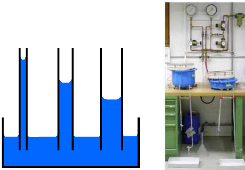
Abbildung 9: Kapillare Saugspannung in Abhängigkeit des Durchmessers der Kapillare (links) und Messung der Saugspannung im Laborversuch (rechts, Quelle: IBP)
