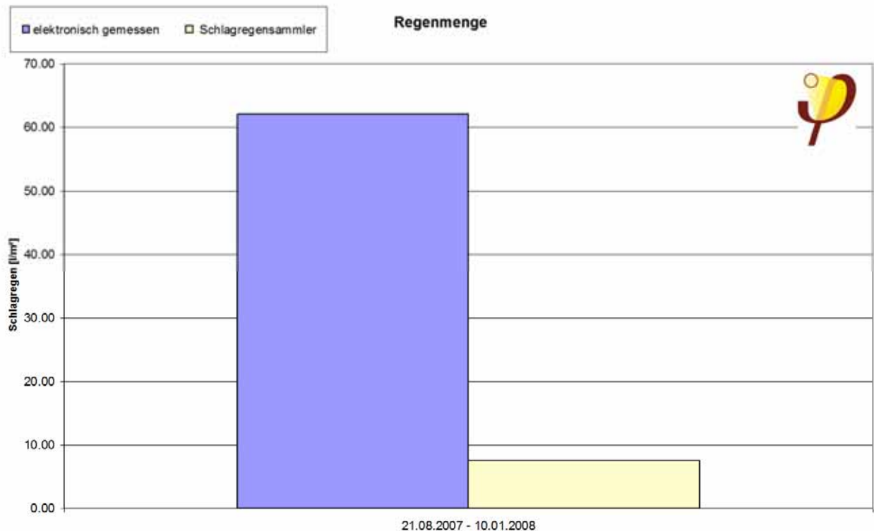
Abbildung 7.: Vergleich der Schlagregenmengen aus elektronischer Messung und Schlagregensammler
