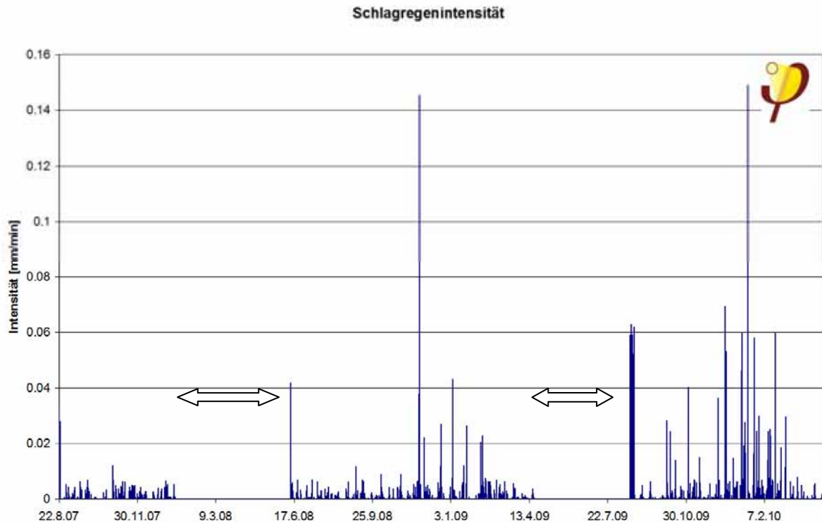
Abbildung 4. Aufgezeichnete Regenereignisse, Perioden ohne Regensignal
