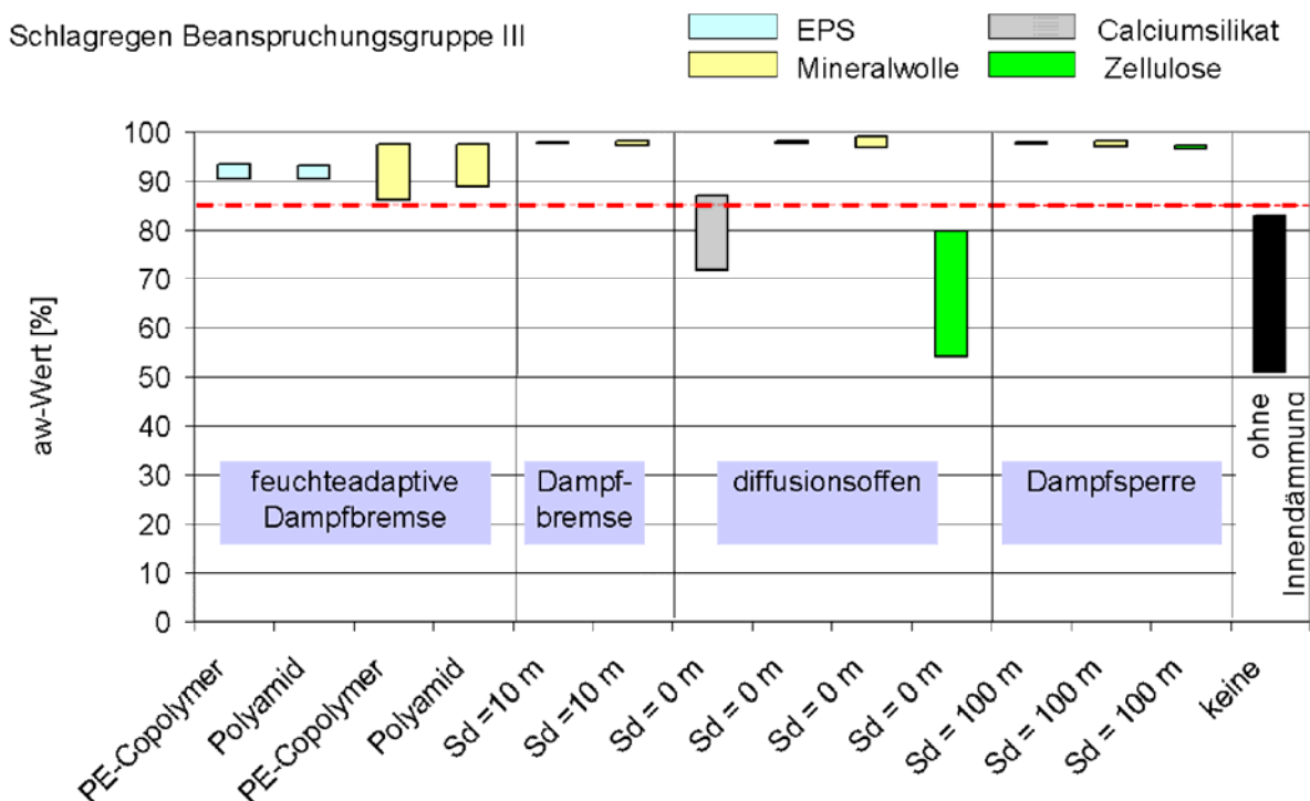
Ergebnisübersicht der aw-Werte; Außenwand westorientiert, ohne wasserabweisende Fassadenbeschichtung, Schlagregen Beanspruchungsgruppe III (aus AkkP 32)
