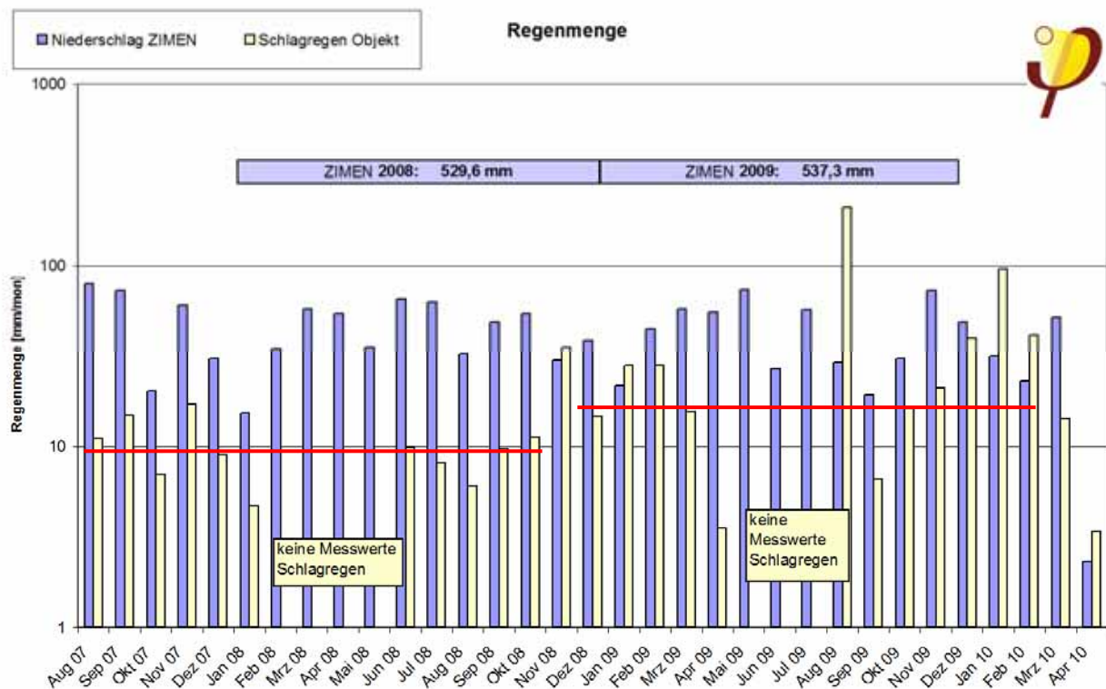
Abbildung 5. Übersicht Regenmengen (logarithmische Darstellung); Vergleich der Schlagregenmessung an der Fassade und der Niederschlagsmengen der Station Neuwied-Hafenstraße [ZIMEN], für die auch die jährlichen Gesamtmengen ermittelt wurden.
