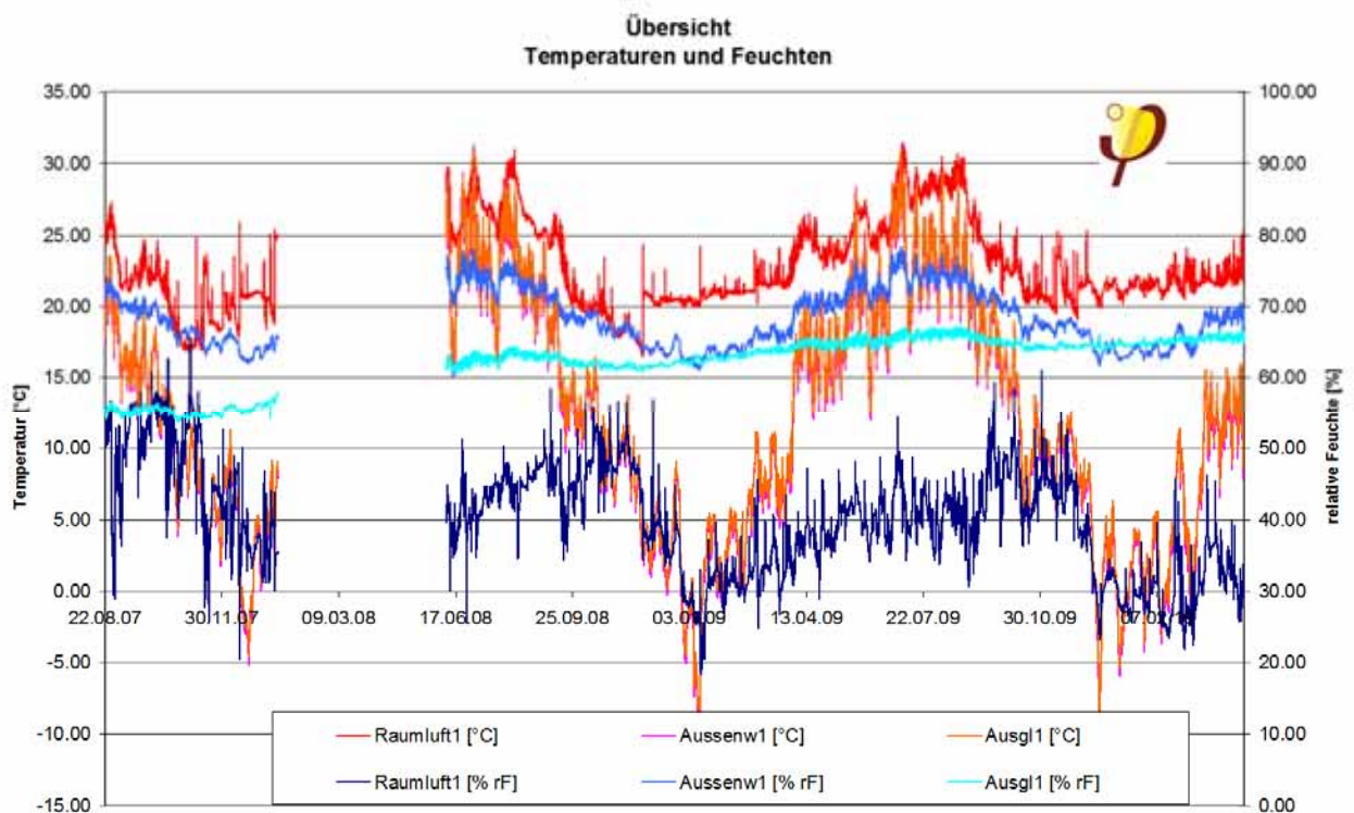
Abbildung 16. Stundenwerte gemessener Ausgleichsfeuchten in verschiedenen Bauteilschichten, der zugehörigen Temperaturen sowie Raumlufttemperatur
