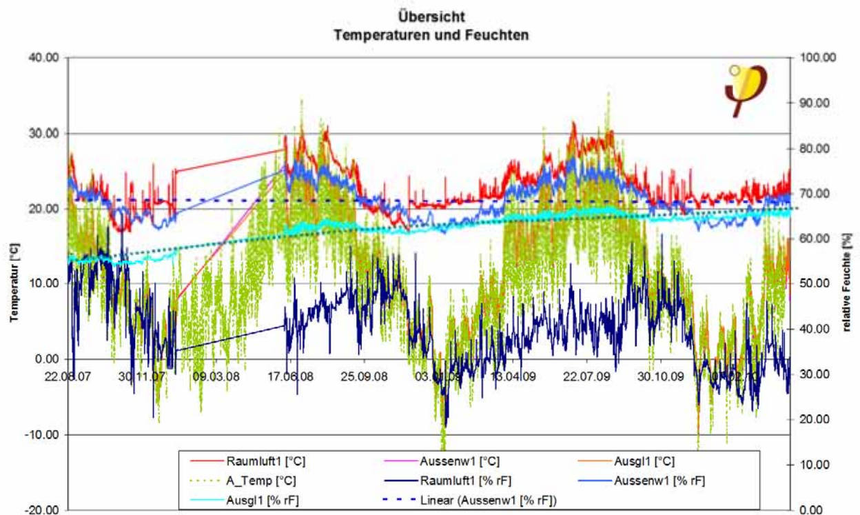
Abbildung 19. Messwerte der Wasseraktivität des ausgeführten Wandaufbaus mit Ausgleichsschicht zwischen Beton und VIP-Innendämmung; hellblaue Kurve: Wasseraktivität in der Ausgleichsschicht
