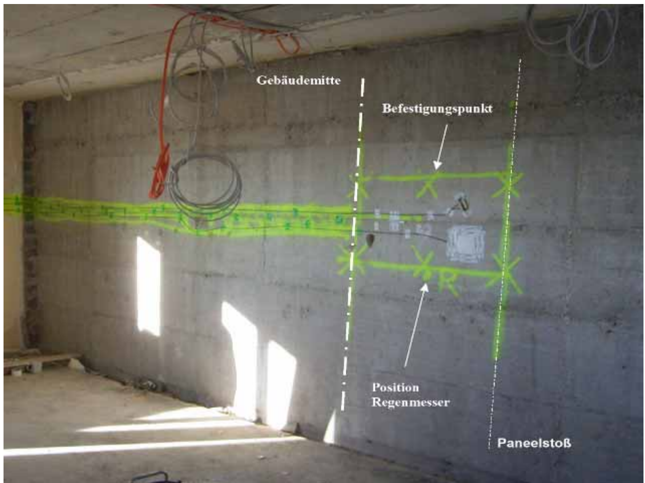
Abbildung 2. Sensorfeld an der Innseite der Außenwand während der Bauarbeiten
