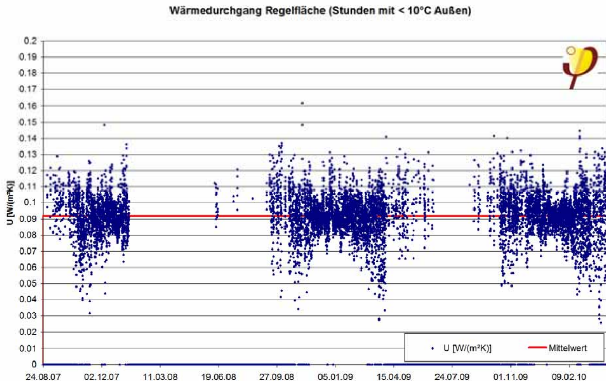
Abbildung 23. Aus den gemessenen Wärmeströmen und Temperaturdifferenzen berechnete Wärmedurchgangskoeffizienten (blau) und das arithmetische Mittel (rot)
