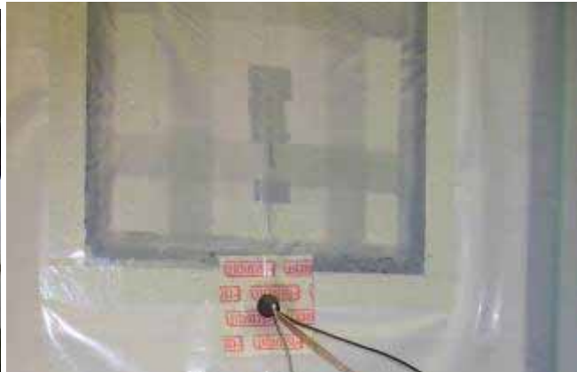
Abbildung 21: Einbaurahmen mit Folienkaschierung und eingebauter Probe inkl. Kabeldurchführung
