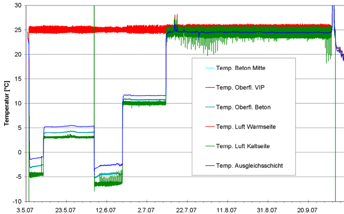
Abbildung 28: Temperaturverläufe in Klimakammer und am Probenkörper
