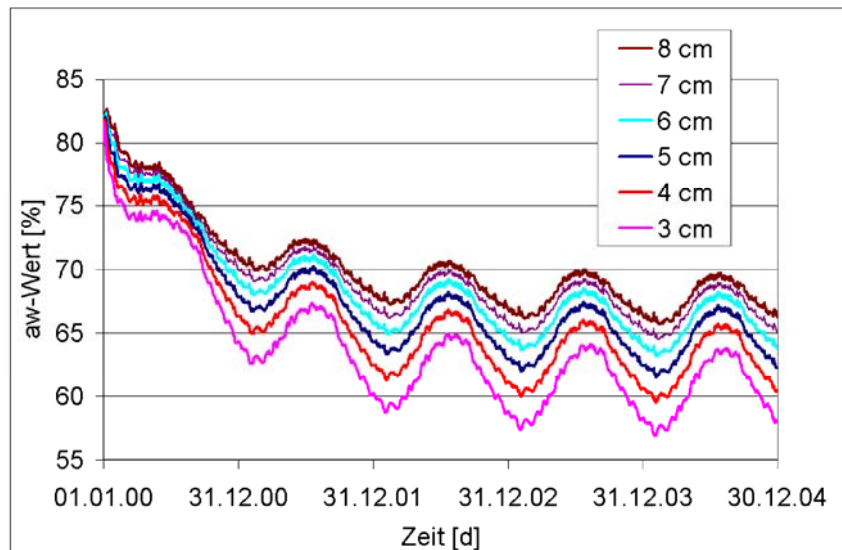
Abb. Feuchteverhalten im Bereich des Innenputzes auf dem Bestandsmauer (aw-Wert) bei EPS-Innendämmung unterschiedlicher Dämmstärke (von 3 bis 8 cm) mit Dampfsperre; wasserabweisende Fassadenbeschichtung, Schlagregengruppe III, Berechnungen mit DELPHIN (Institut für Bauklimatik IBK, TU-Dresden) [PHI 2006]
