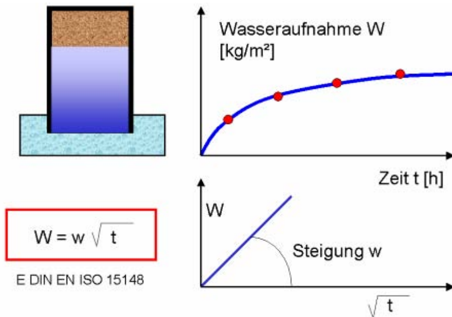
Abbildung 10: Bestimmung des Wasseraufnahmekoeffizienten w mittels Saugversuch und Auswiegen
