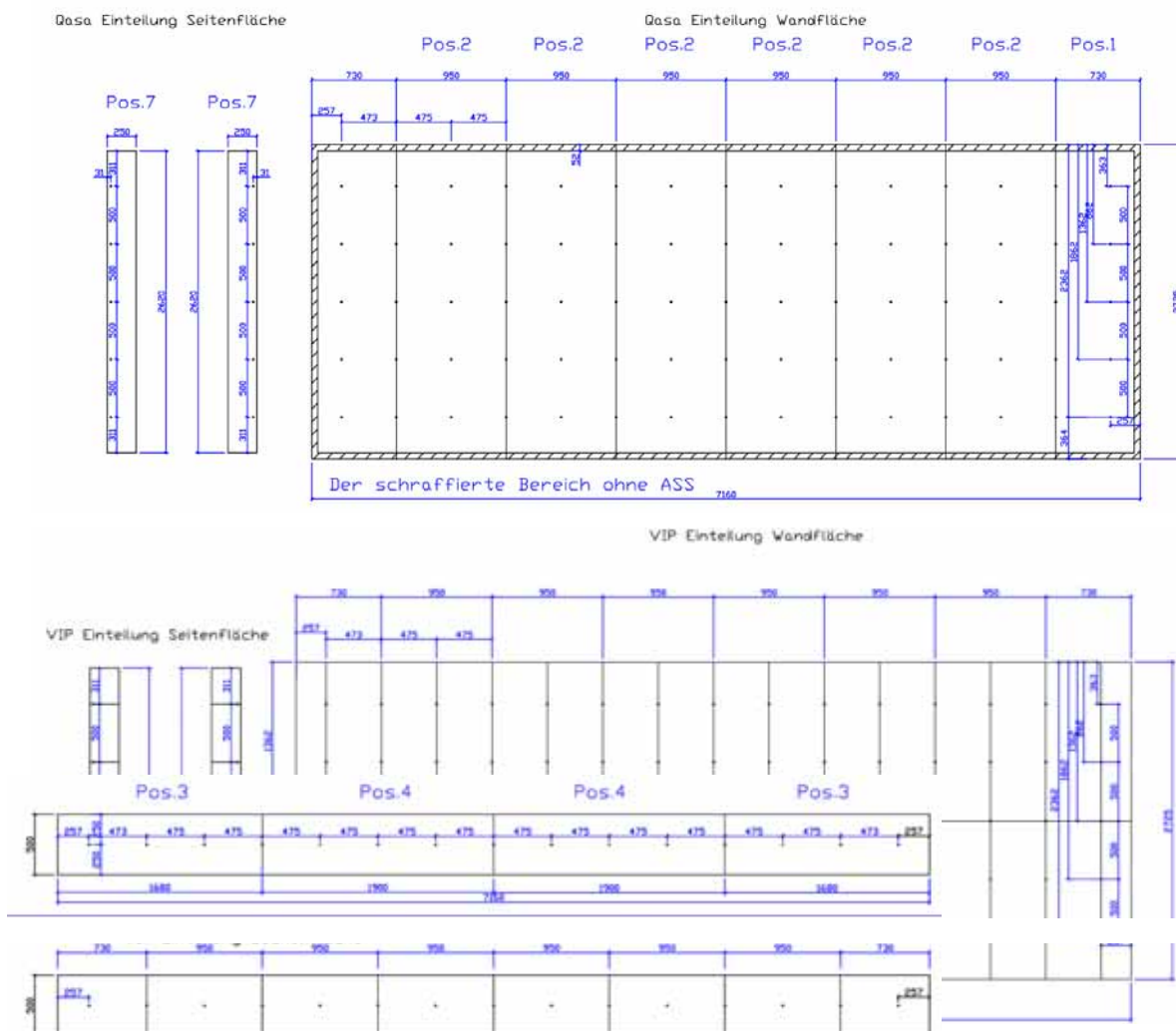
Pilotobjekt Neuwied Paneeleinteilung und innere VIP-Einteilung der Begleitdämmung an Decke und Boden
