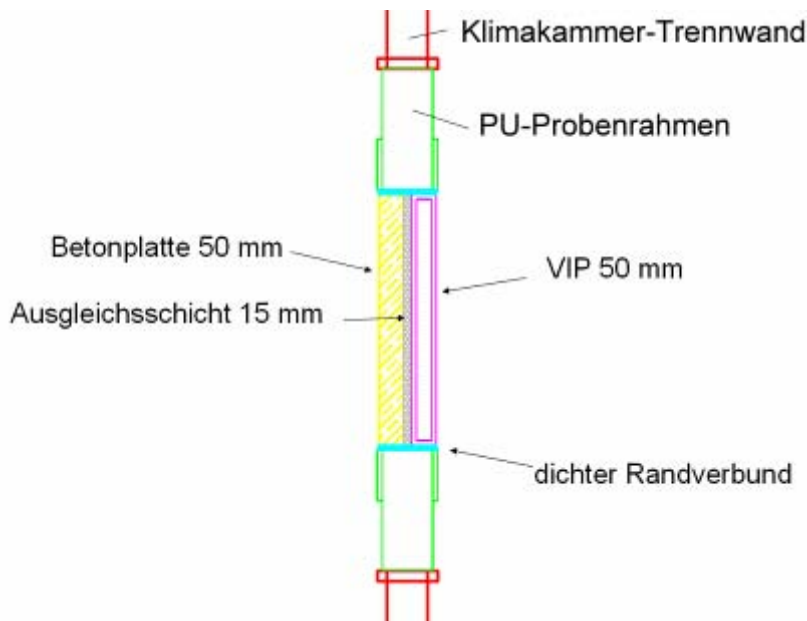
Abbildung 15 Schichtaufbau des Probenkörpers
