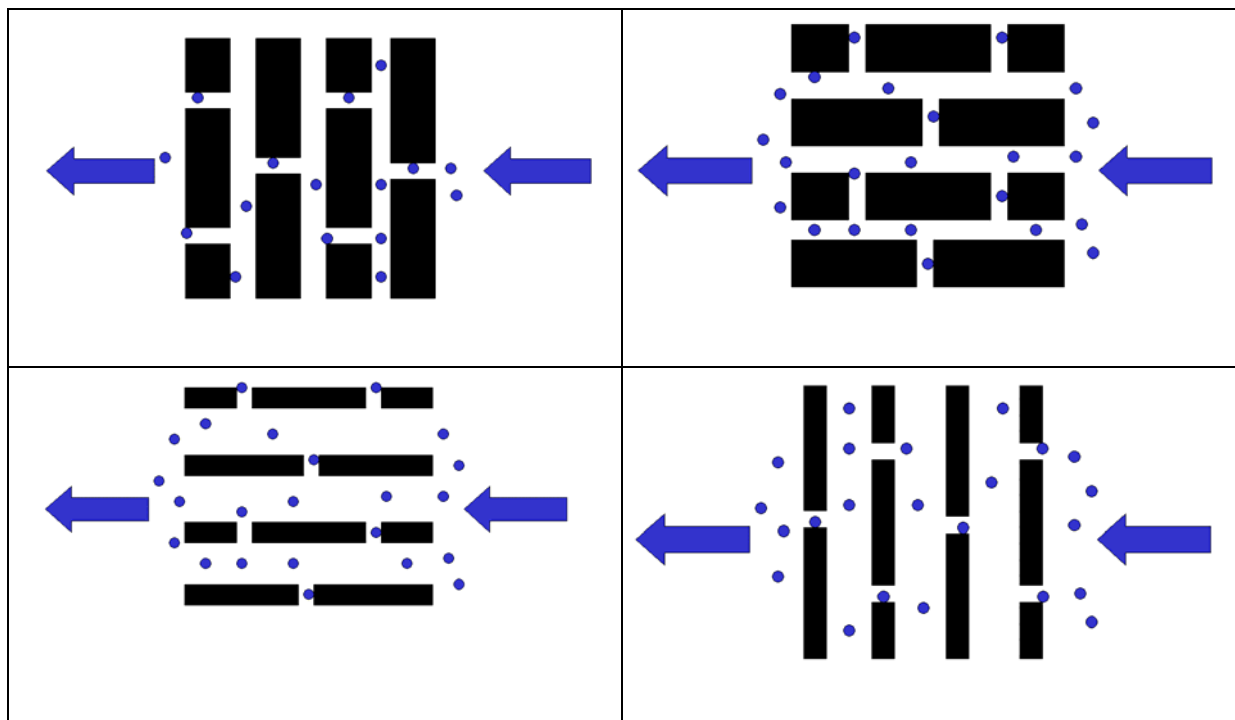
Abbildung 7: Diffusion durch Materialien unterschiedlicher Porosität und Porengeometrie
