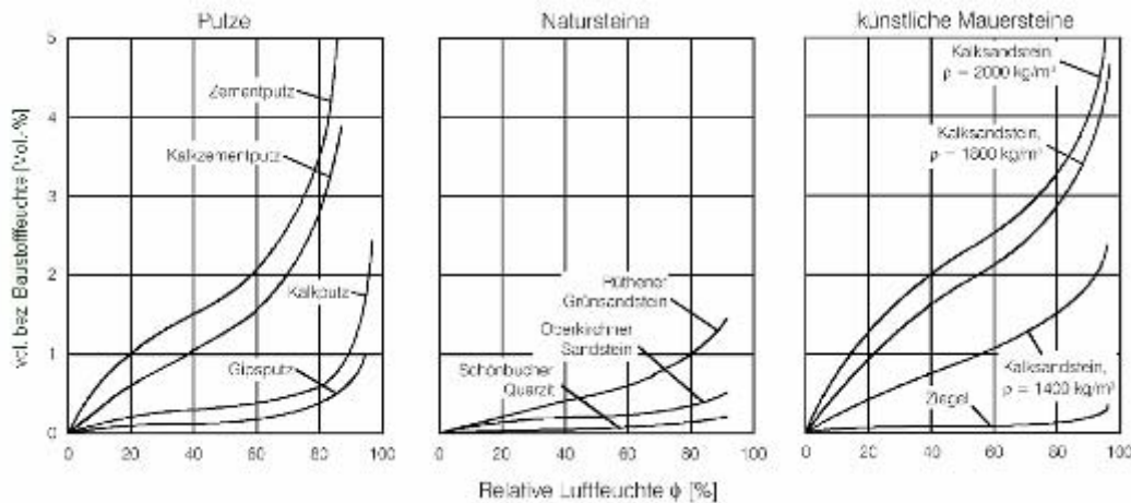
Abbildung 3: Sorptionsisothermen unterschiedlicher Baustoffe (nach [Künzel 94])
