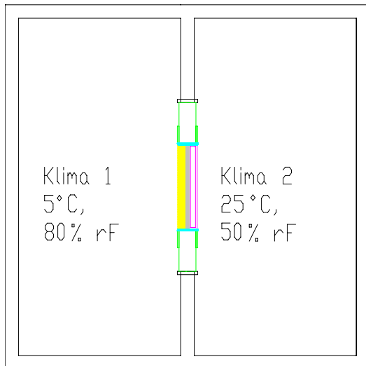
Abbildung 19: Differenzklimakammer-Prüfstand (Klima 1: „Außenklima bzw. Kaltseite“, Klima 2: „Innenklima bzw. Warmseite“)
