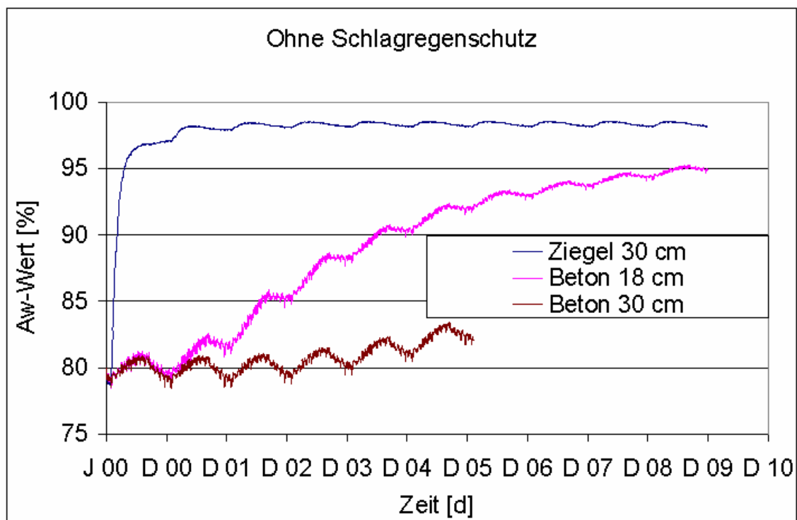
Abbildung 13: Verlauf der Wasseraktivität an der Innenoberfläche des Wandaufbaus ohne Schlagregenschutz bei unterschiedlichen Wandbildnern (Beton 18 cm, Beton 30 cm und Ziegel 30 cm)
