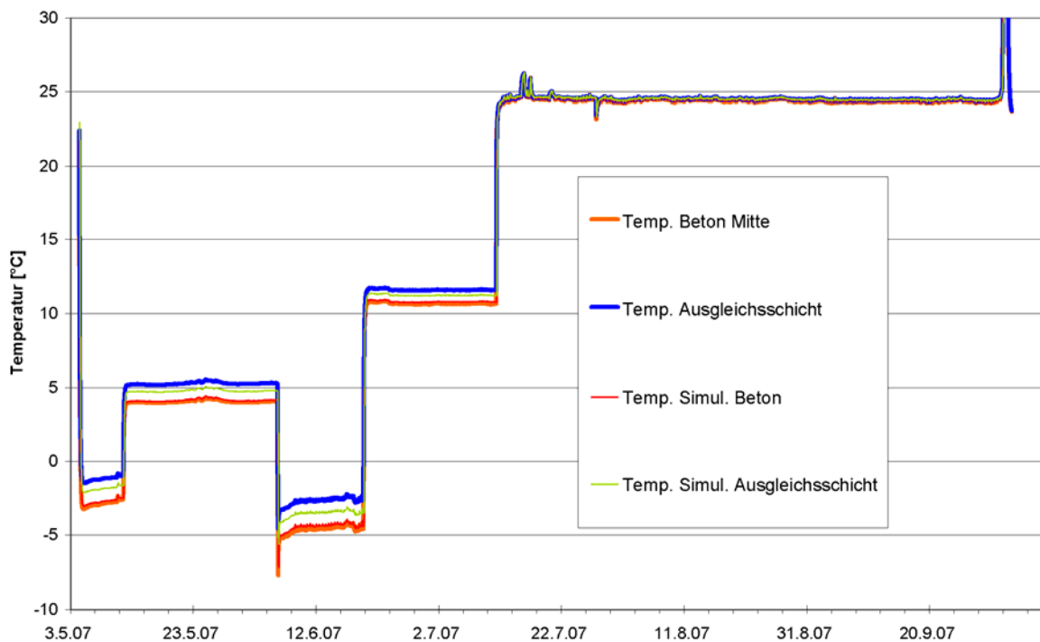
Abbildung 32: Vergleich der gemessenen und berechneten Temperaturverläufe im Beton und in der Ausgleichsschicht
