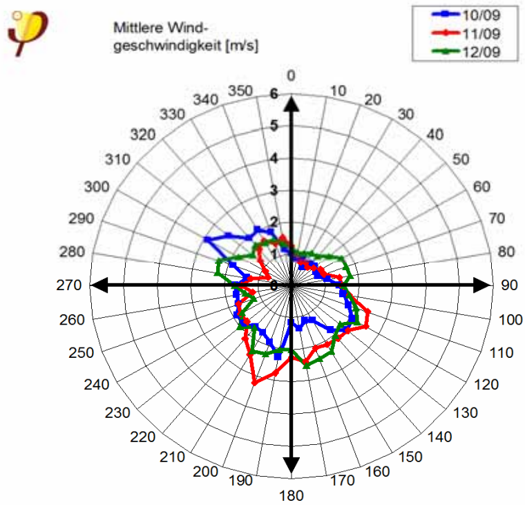
Anhang A 10: Polardiagramm Wind 4. Quartal 2009
