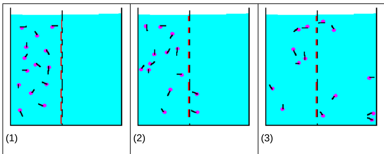
Abbildung 6: Diffusion als Konzentrationsausgleich durch thermische Eigenbeweglichkeit
