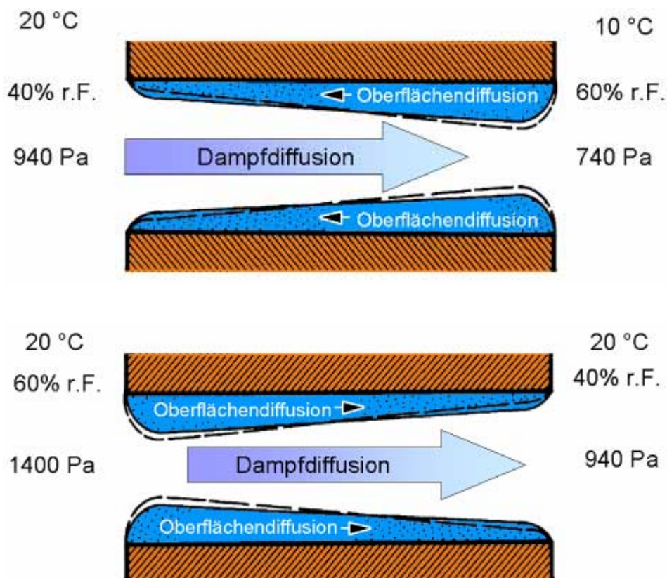
Abbildung 8: Transportrichtung von Wasserdampfdiffusion und Oberflächendiffusion in Abhängigkeit von Wasserdampfpartialdruck und relativer Feuchte; je nach Randbedingung können die Transportrichtungen gegen- oder gleichgerichtet sein.
