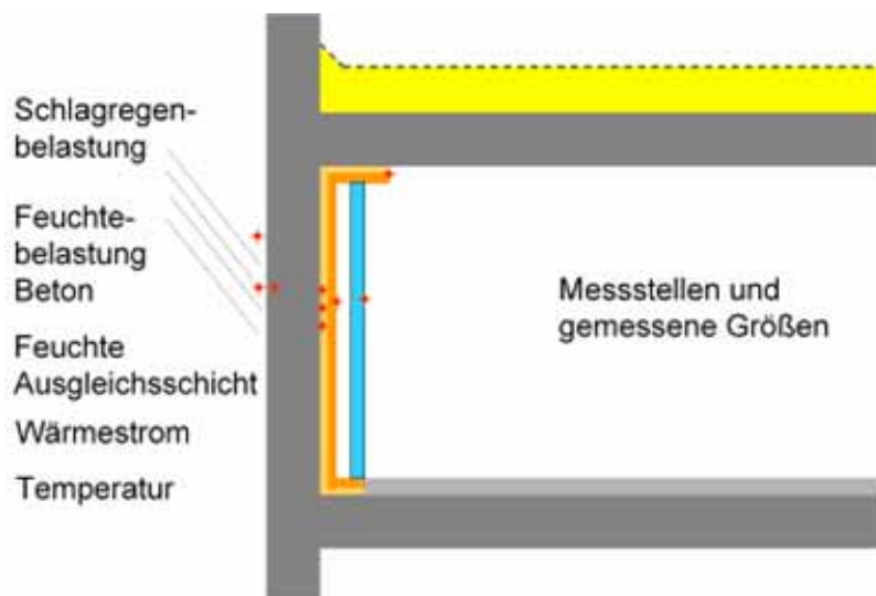
Abbildung 1. Übersicht Messstellen
