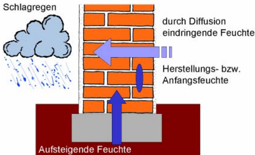
Abbildung 1: Feuchtequellen bei Außenwänden (Beregnung, Tauwasseranfall, aufsteigende Grundfeuchte und anfängliche Baufeuchte)
