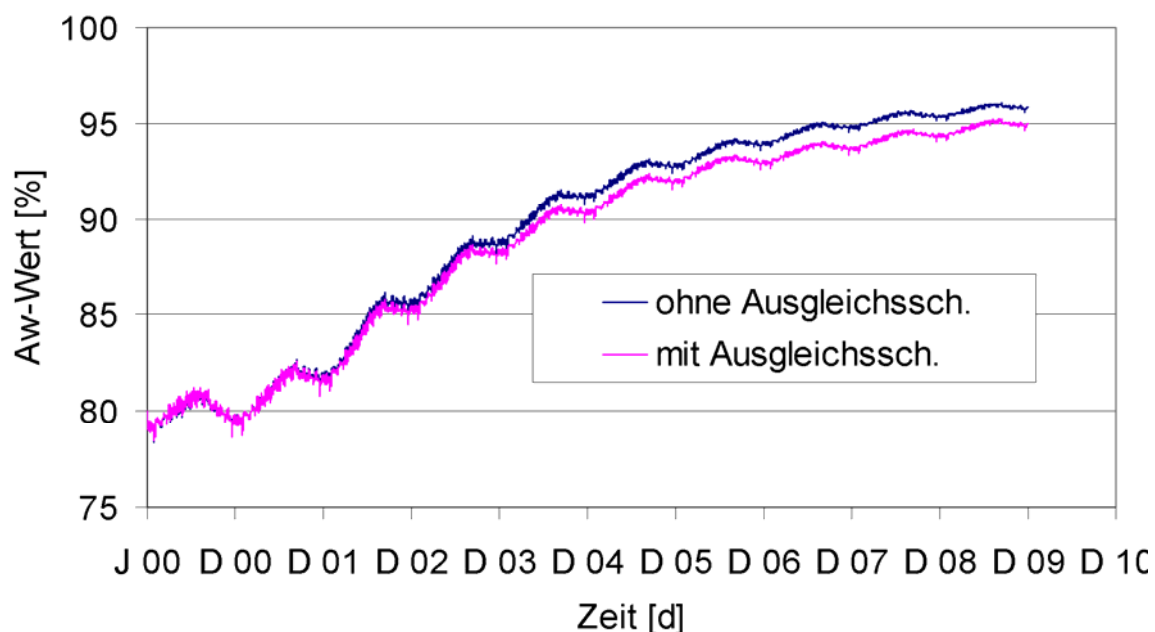
Abbildung 11: Verlauf der Wasseraktivität des Wandaufbaus ohne Anstrich und Spachtelung jeweils mit und ohne Ausgleichsschicht zwischen Beton und VIP-Innendämmung
