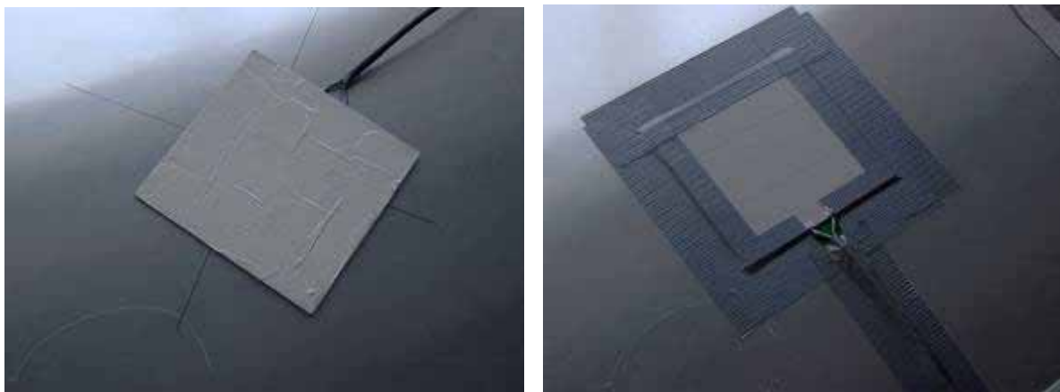
Abbildung 24 Wärmeflussmessplatte auf dem VIP-Element
