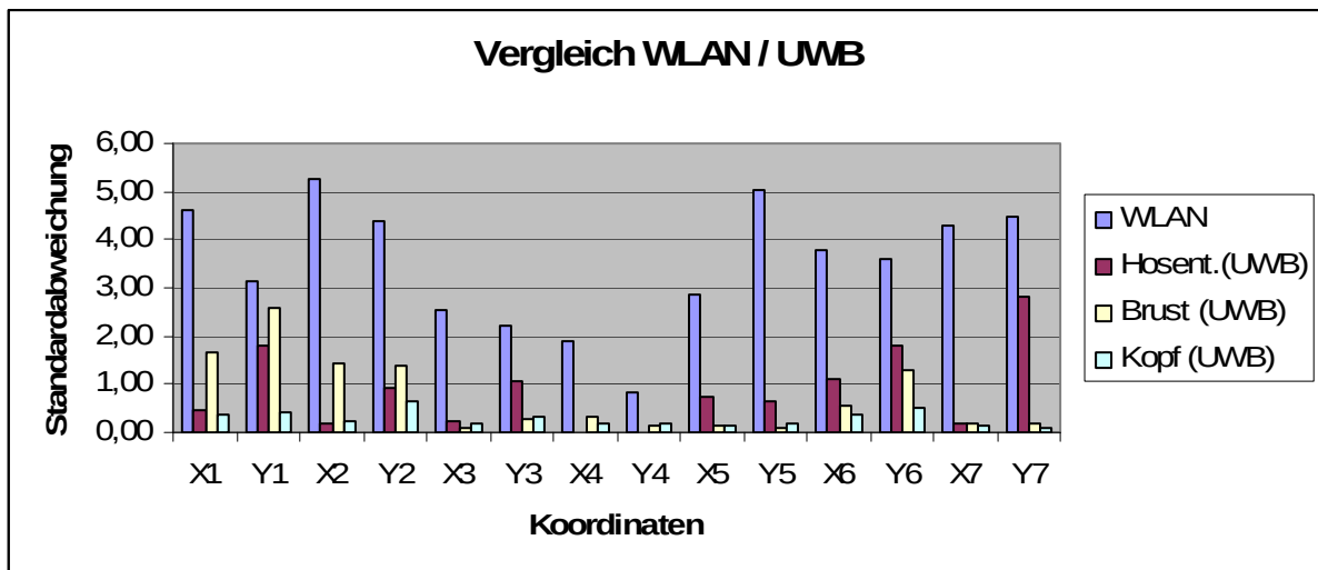
Abbildung 97: Vergleich WLAN und UWB
