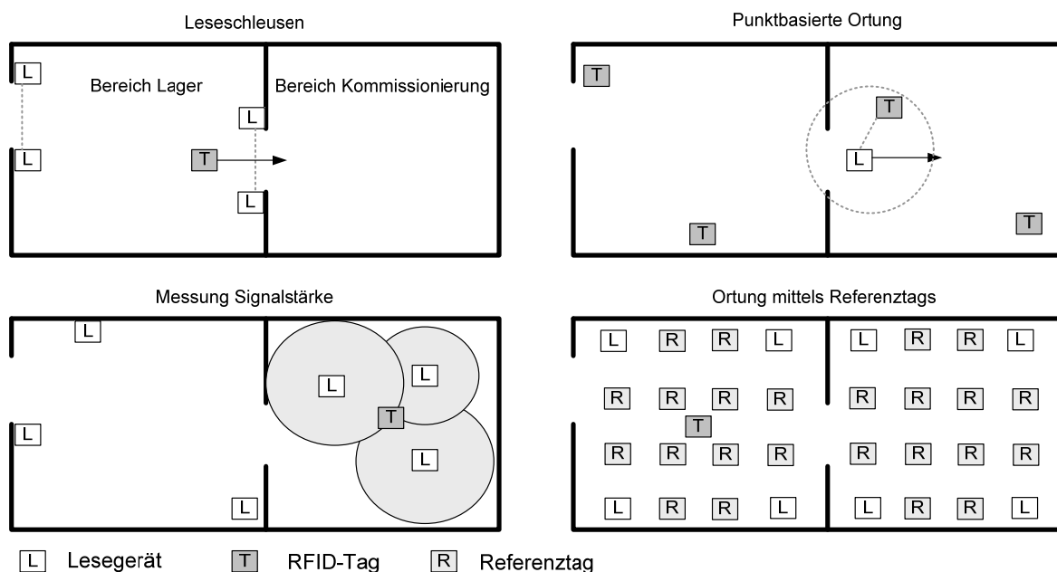
Abbildung 20: Ortung mit RFID-Tags nach [TFH Wildau, 2009]
