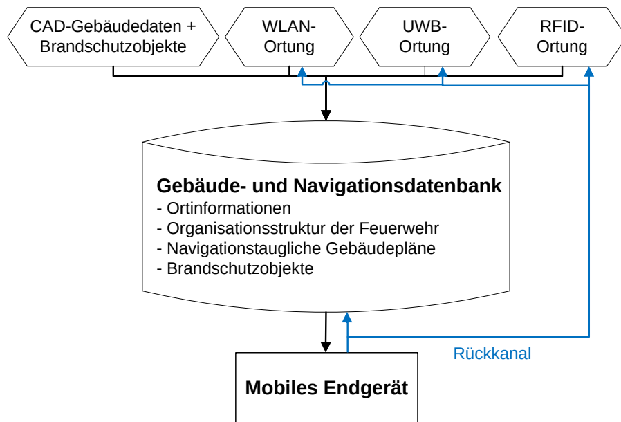
Abbildung 42: Systementwurf Indoor-Navigations-Integrationsplattform
