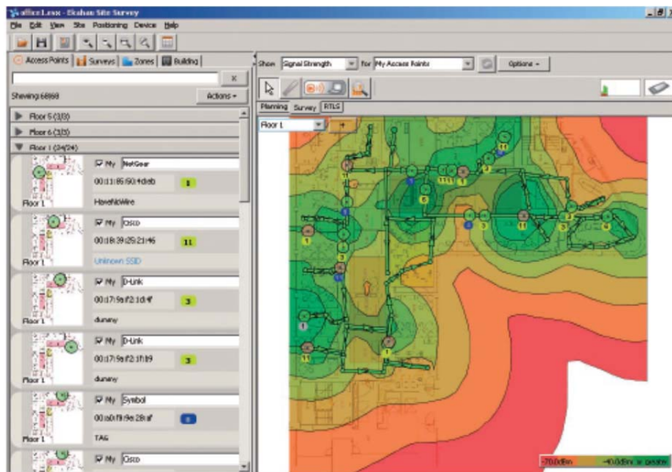
Abbildung 12: Ekahau Site-Survey zur Analyse der Signalstärken [Ekahau, 2009]
