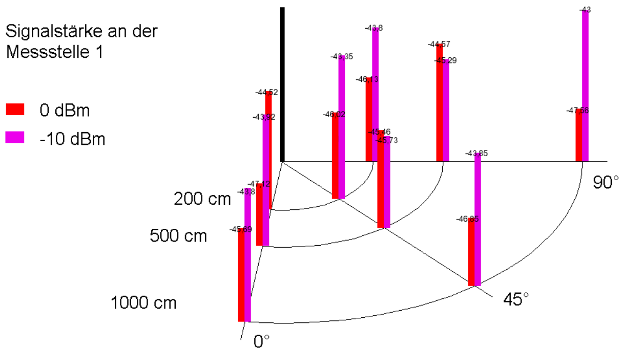
Abbildung 82: Signalstärke an Messstelle 1
