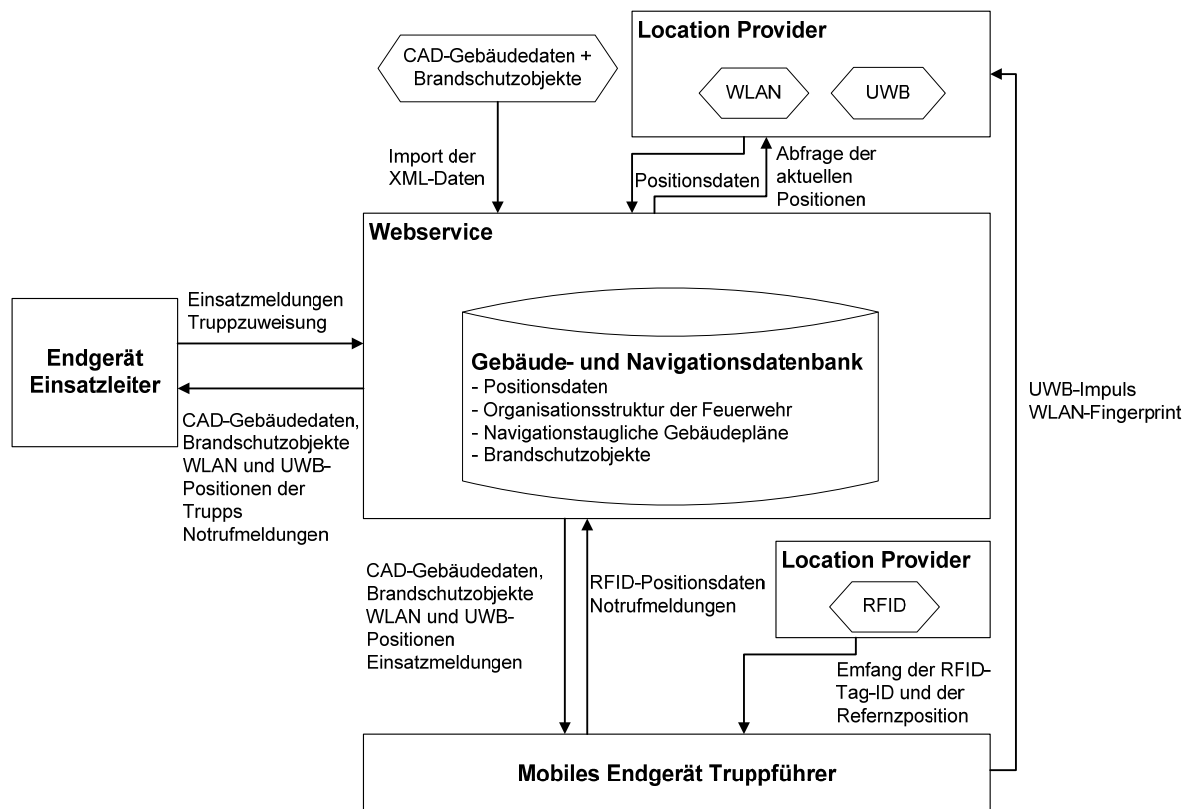
Abbildung 54: Systemkomponenten der INI
