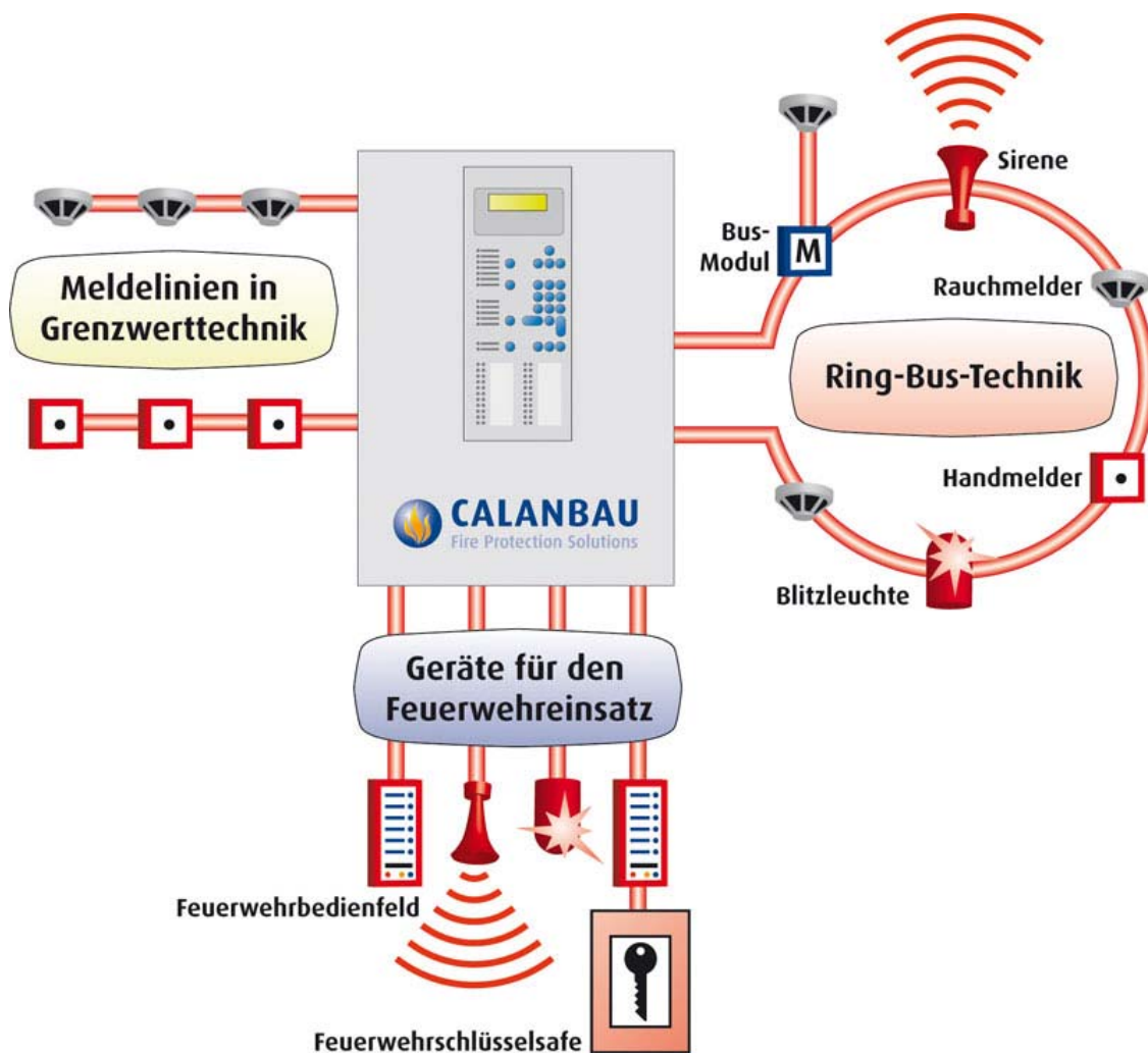
Abbildung 29: Aufbau einer Brandmeldeanlage
