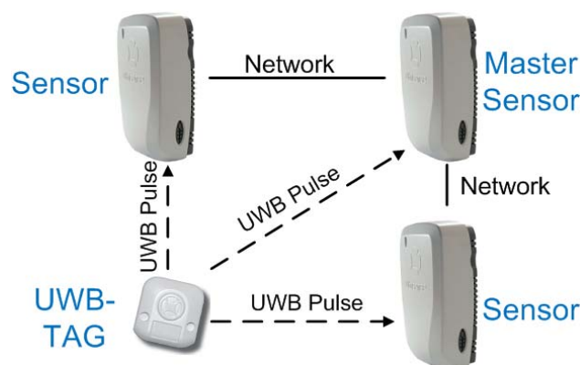
Abbildung 13: Ubisense UWB-System nach [Becker, 2008]
