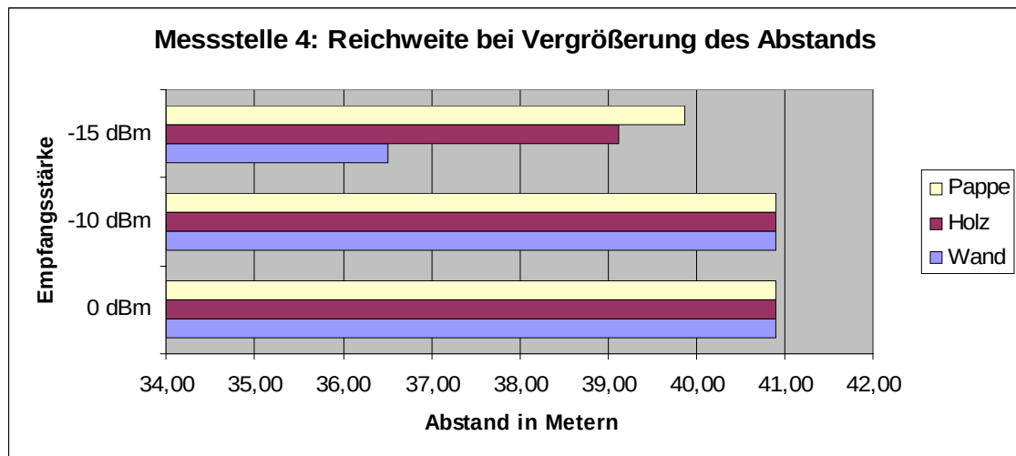
Abbildung 87: Reichweite bei Vergrößerung des Abstandes (Messstelle 4)
