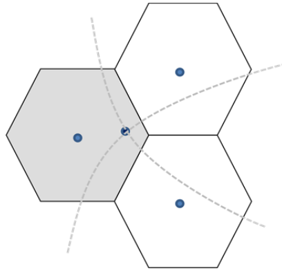
Abbildung 4: Time Difference of Arrival nach [Télématique, 2009]
