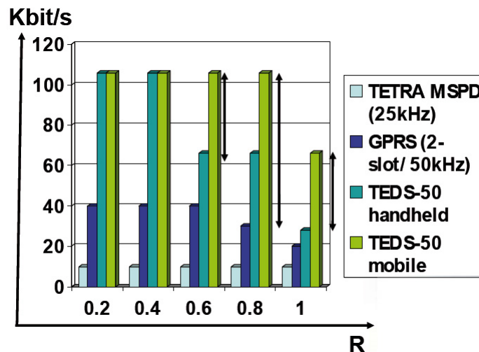
Abbildung 39: Datenraten BOS-Funk [Kaszynski, 2008]
