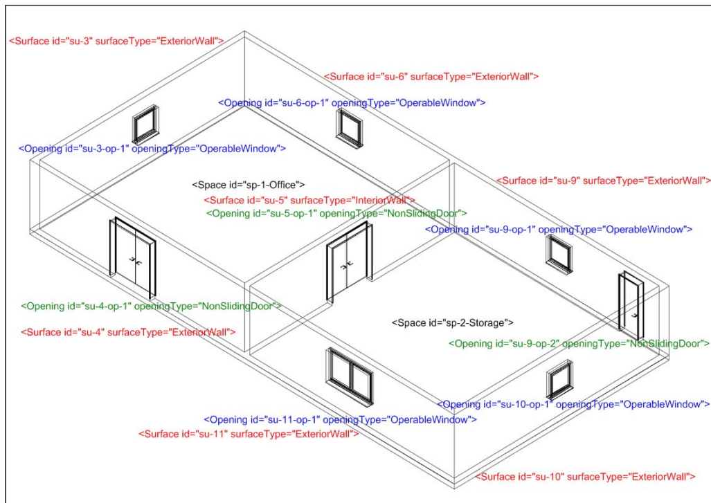
Abbildung 45: 3D-Gebäudemodell und gbXML-Elemente [Schatz, 2008]
