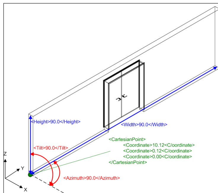
Abbildung 46: RectangularGeometry Modell [Schatz, 2008]
