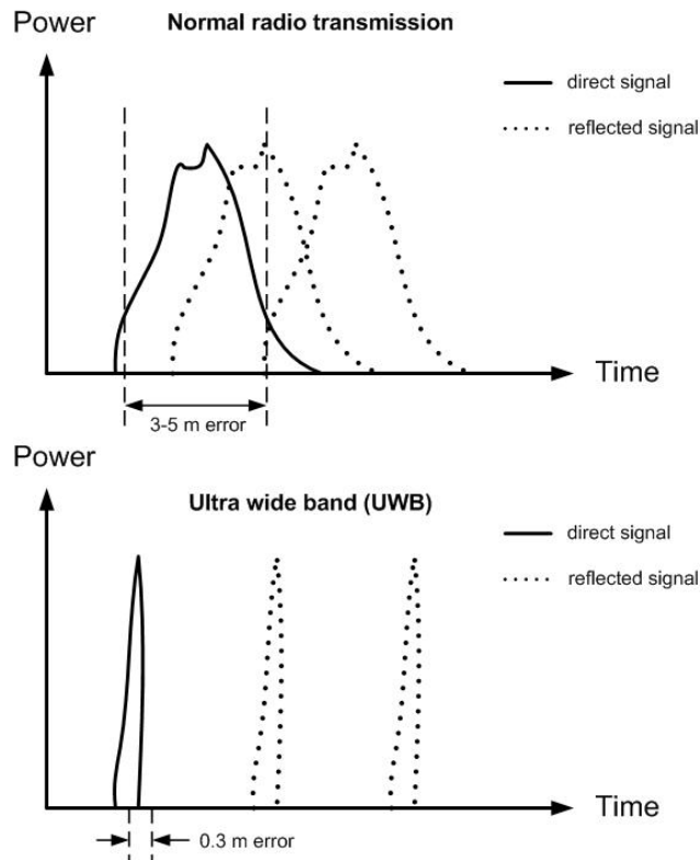
Abbildung 21: Signalausbreitung Konventionelle Funktechnologie und UWB nach [Becker, 2008]
