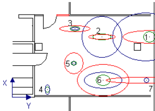
Abbildung 90: UWB-Messung: Darstellungen der Standardabweichungen
