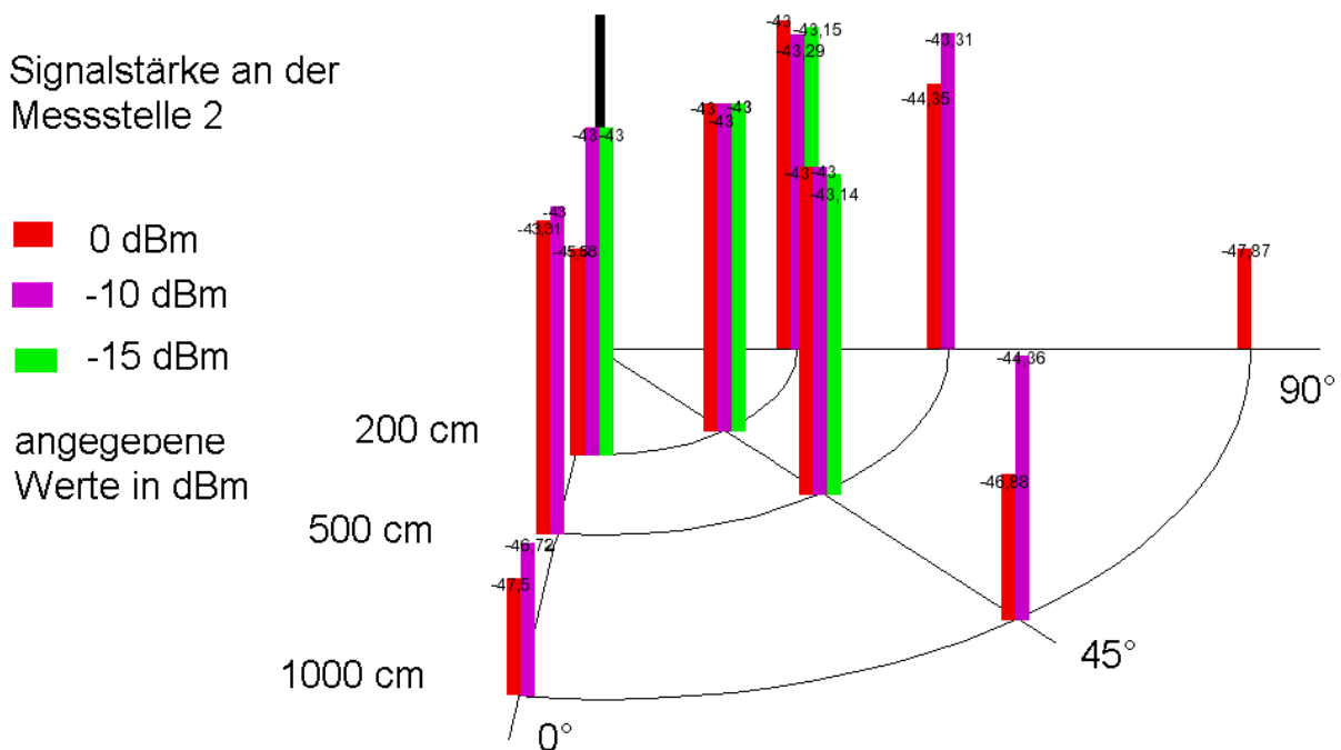
Abbildung 83: Signalstärke an Messstelle 2
