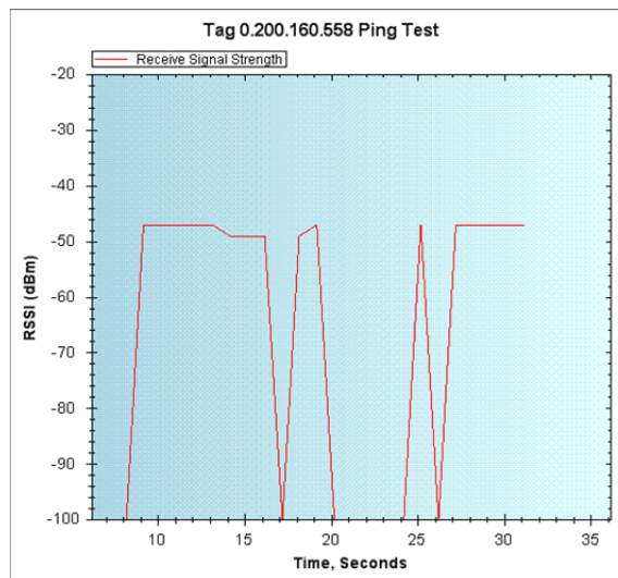
Abbildung 79: Diagramm zur Messung der Signalstärke
