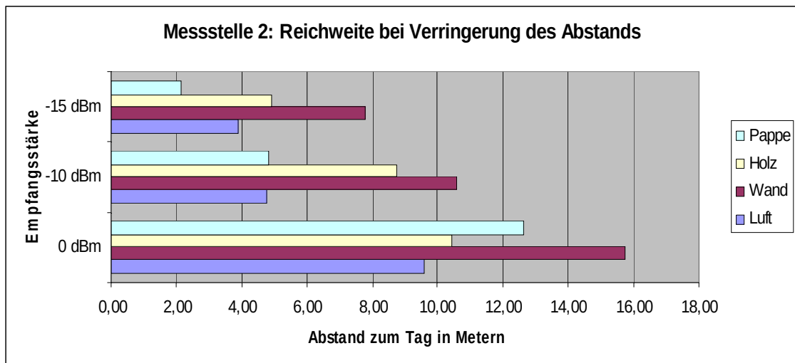
Abbildung 84: Reichweite bei Verringerung des Abstands (Messstelle 2)
