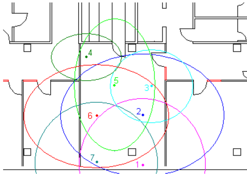
Abbildung 96: WLAN-Messung: Darstellung der Standardabweichungen im Computerlabor
