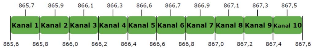
Abbildung 18: Kanalaufteilung, Quelle: [Füßler & Clasen, 2005]
