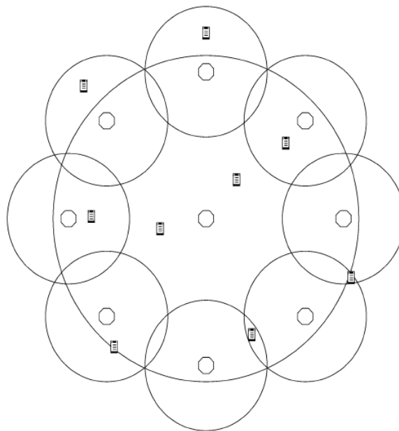
Abbildung 8: Landmark: Aufbau mit 9 Readern mit zwei unterschiedlichen Reichweiten [Ni, Liu, Lau, & Patil, 2003]
