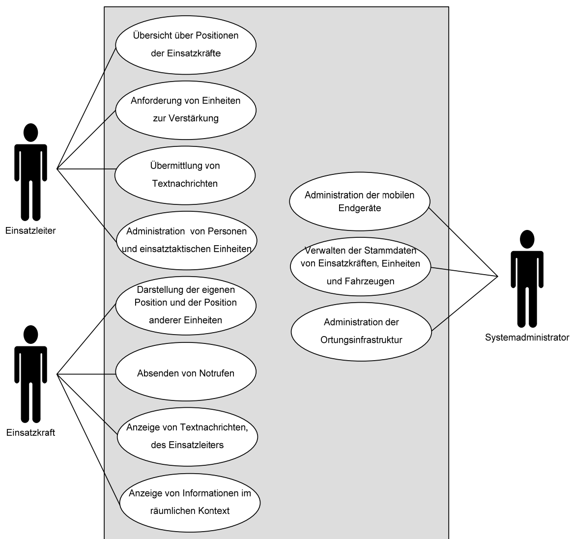
Abbildung 41: Use Case-Diagramm
