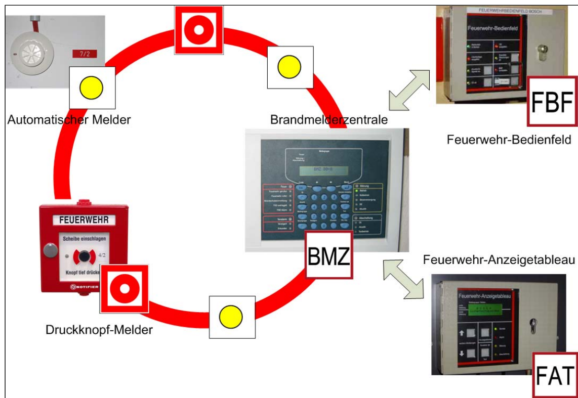
Abbildung 43: Aufbau einer Brandmeldeanlage / Symbolik für den Einsatzablauf [Schatz, 2008]
