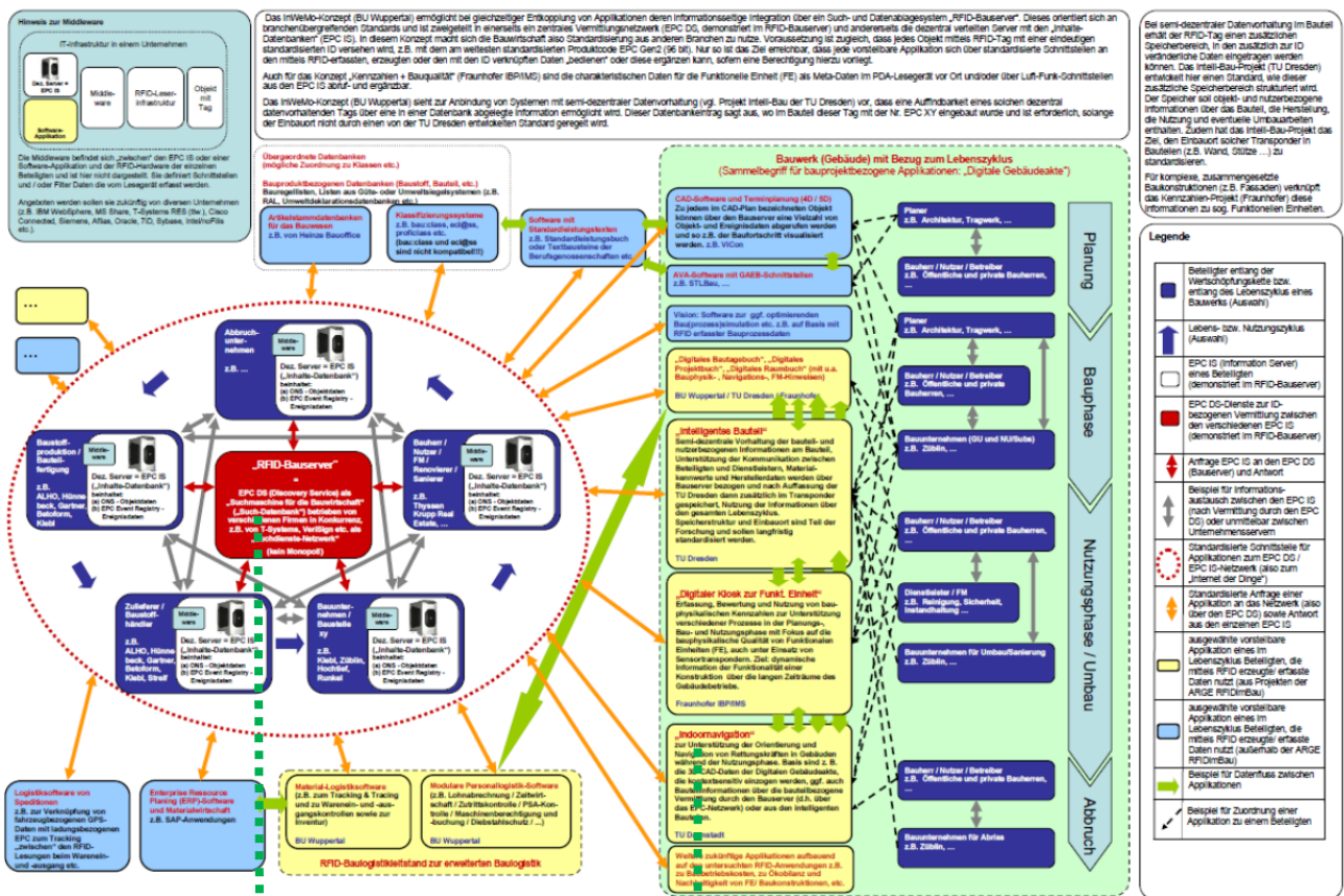
Abbildung 99: Schnittstellübersicht innerhalb der ARGE RFIDimBau, siehe www.rfidimbau.de
