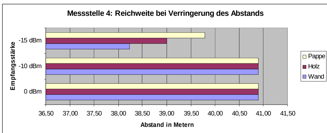
Abbildung 86: Reichweite bei Verringerung des Abstands (Messstelle 4)
