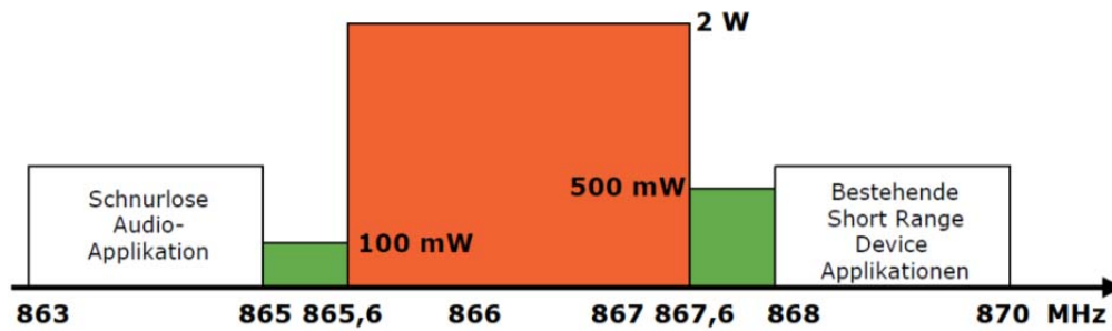
Abbildung 17: UHF Nutzung der Frequenzbereiche [Füßler & Clasen, 2005]:
