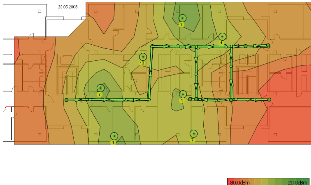
Abbildung 23: Einmessung mit vorgegebenen Wegen mit der Ekahau Sitesurvey
