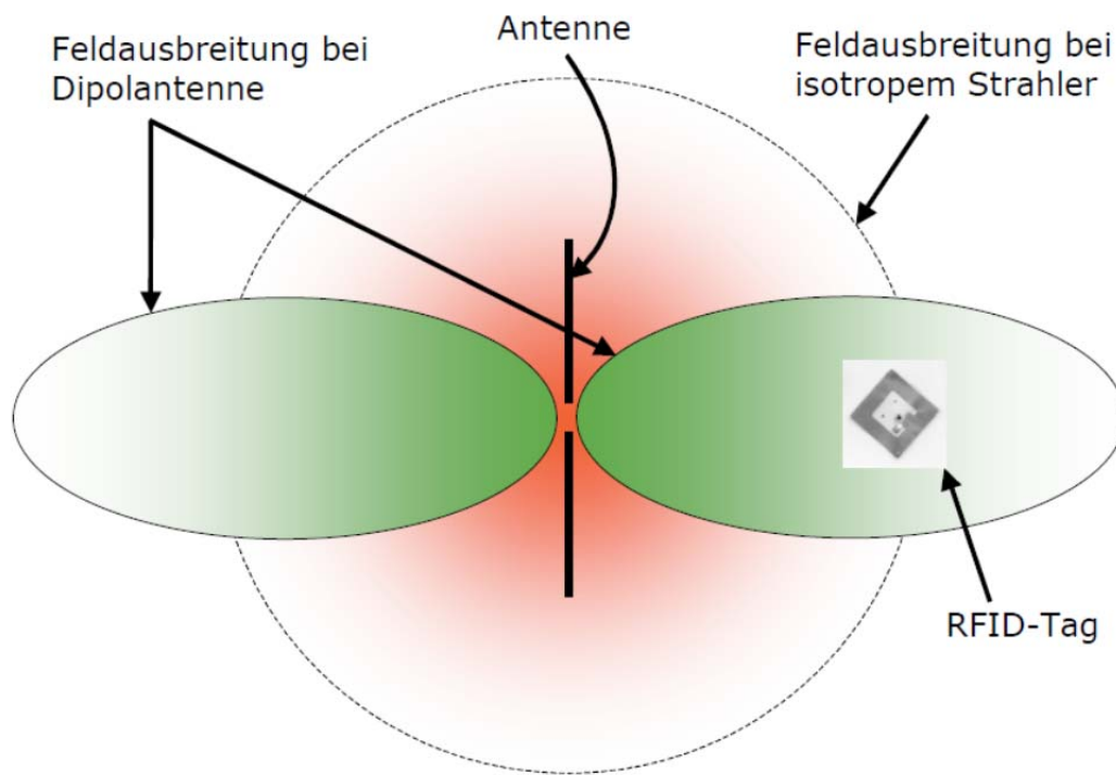
Abbildung 19: Feldausbreitung Isotroper Strahler vs. Dipolantenne, Quelle: [Füßler & Clasen, 2005].
