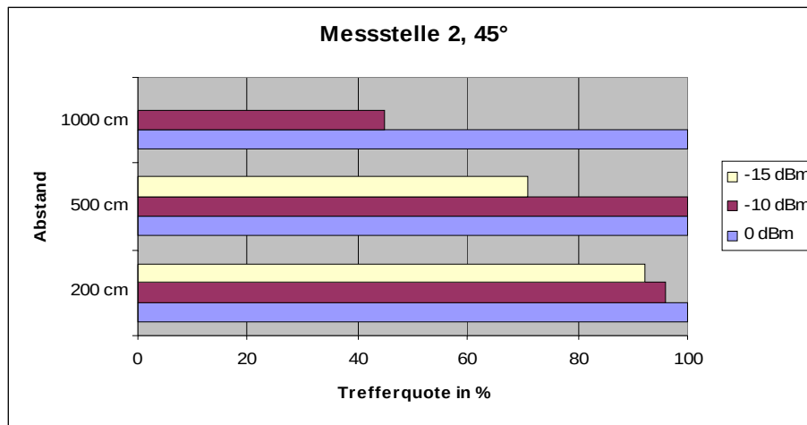
Abbildung 80: Messstelle 2, 45°
