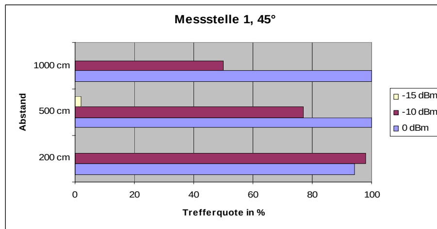
Abbildung 81: Messung im Computerlabor
