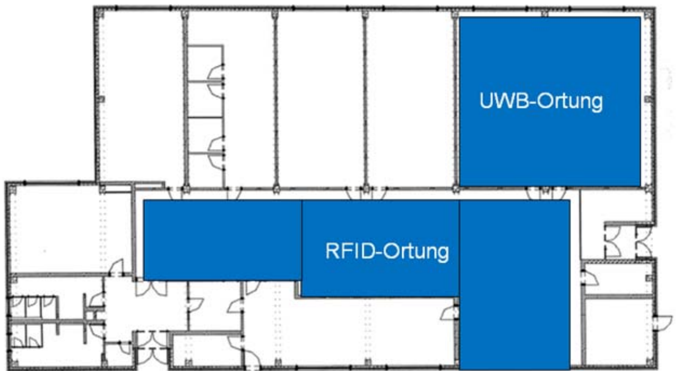
Abbildung 66: Aufbau der Testortungssysteme
