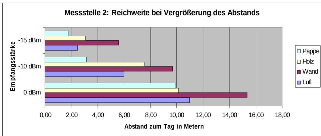
Abbildung 85: Reichweite bei Vergrößerung des Abstands (Messstelle 2)
