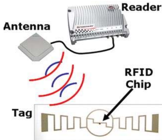
Abbildung 14: Aufbau eines RFID-Systems, (Quelle: http://www.logsystems.hu )
