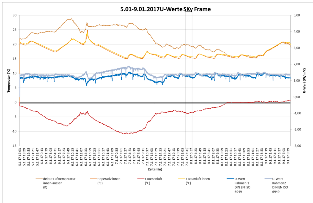
Abbildung 7.13: U-Werte Sky-Frame 5.1.-9.1.2017
