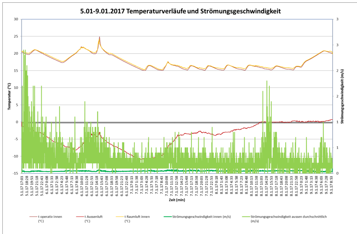
Abbildung 7.9: 5.1.-9.1.2017 Temperaturverläufe und Strömungsgeschwindigkeiten
