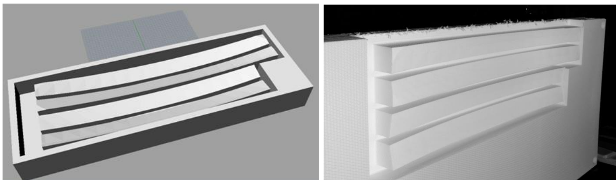
Abbildung 5.18: Screenshot der Formfrästeile zur Einpassung des Pneus in die Hotbox (linkes Bild) und fertig hergestelltes Formfrästeil (rechtes Bild)
