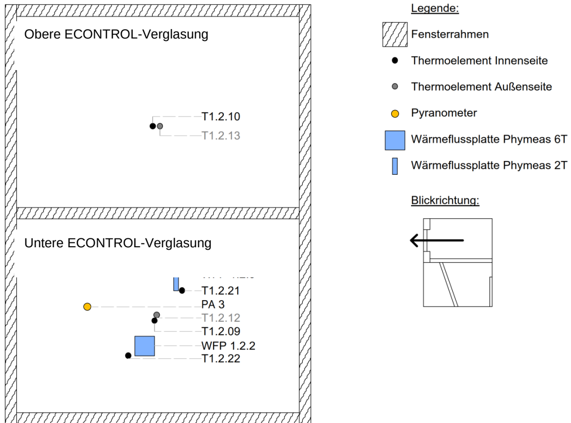
Abbildung 8.4: Sensorik für das Monitoring an der ECONTROL-Verglasung
