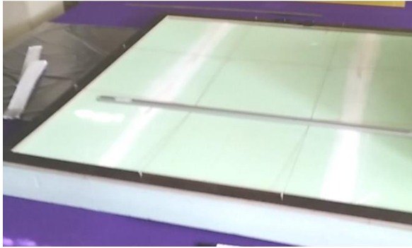
Abbildung 4.6: Positionierung der Rasterschablone (linkes Bild) zur Markierung der Sensorpositionen auf dem Referenzprobekörper (rechtes Bild)
