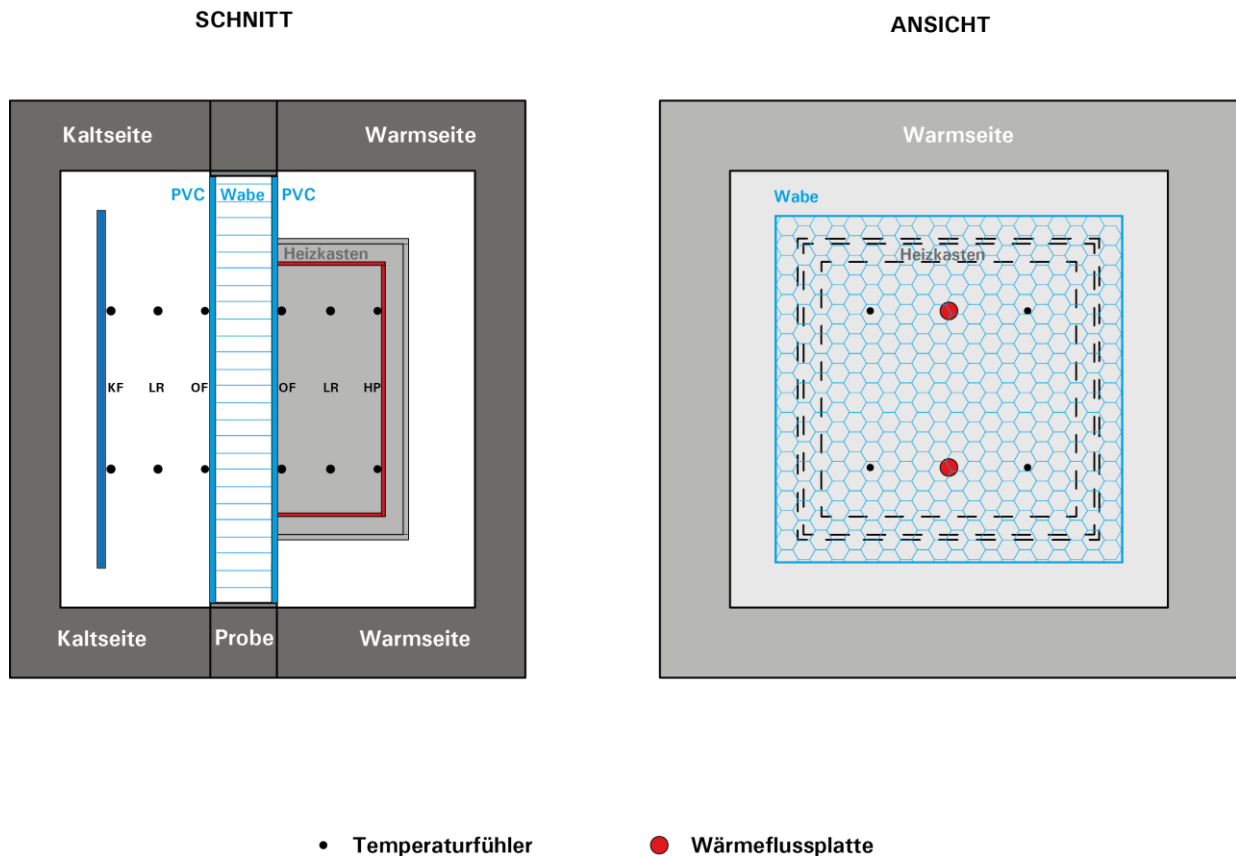
Abbildung 5.11: Versuchsanordnung Wabenaufbau II
