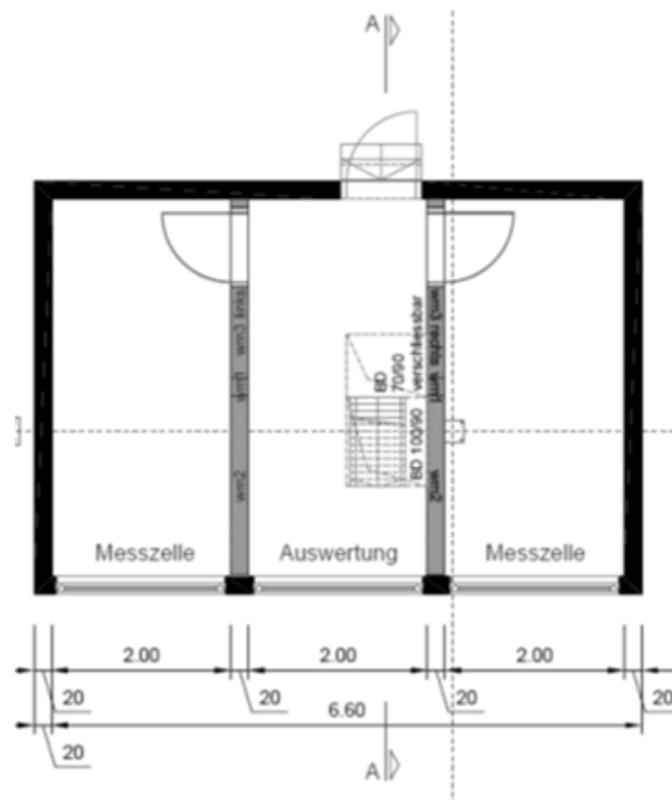
Abbildung 4.39: Grundriss des Fassadenprüfstands im EG (identisch im OG)
