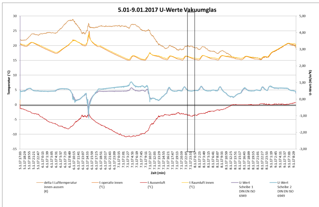
Abbildung 7.10: U-Werte Vakuumglas 5.1.-9.1.2017
