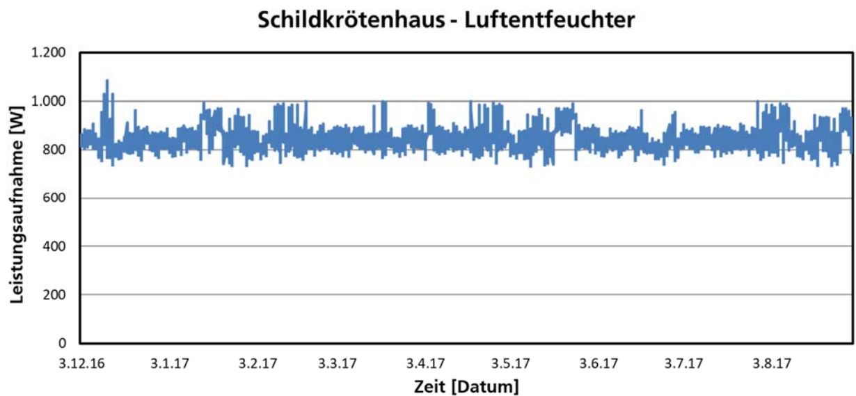
Bild 44: Schildkrötenhaus: Vergleich Leistungsaufnahme Luftversorgung - Luftentfeuchter.
