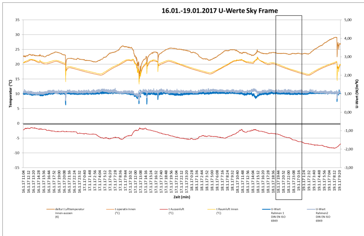
Abbildung 7.20: U-Werte Sky-Frame 16.1.-19.1.2017
