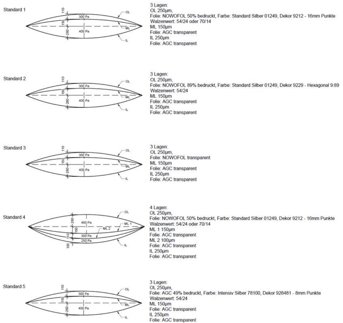
Bild 13: Membran-Prüflinge.
