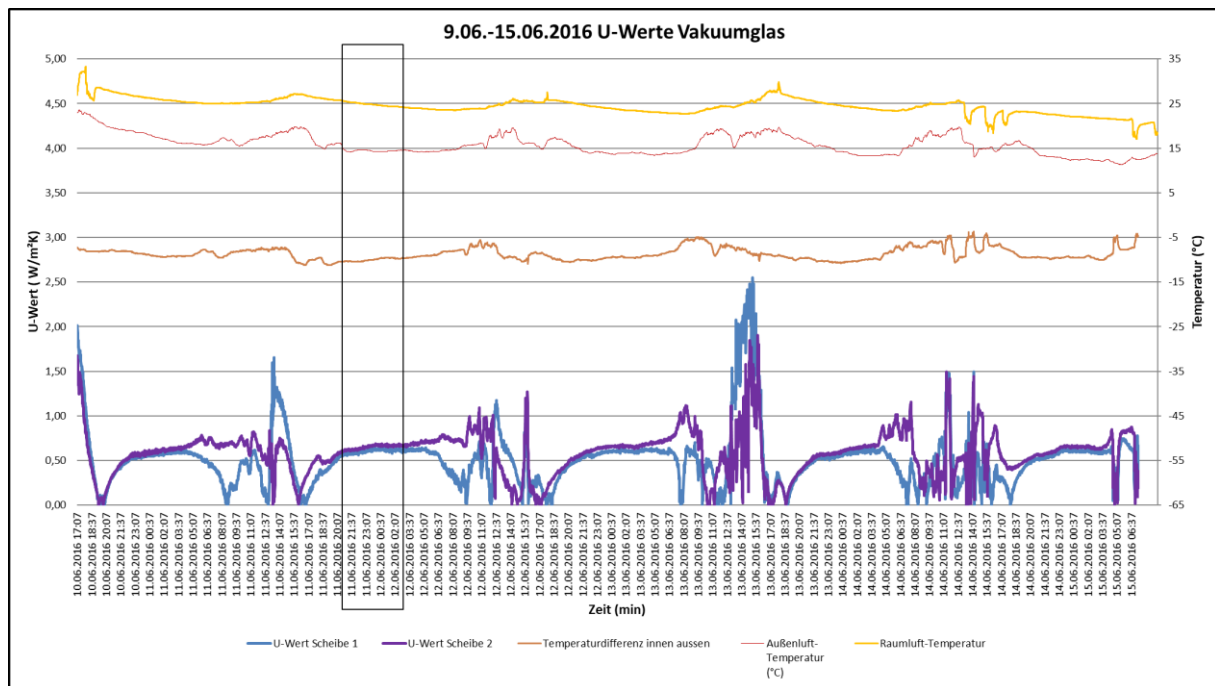
Abbildung 7-23: U-Werte Vakuumglas 9.6.-15.6.2016
