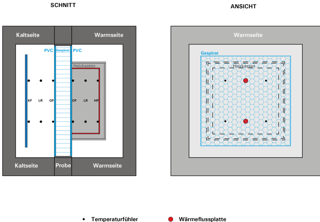
Abbildung 5.13: Versuchsaufbau für die Probe mit Glasfasergespinst
