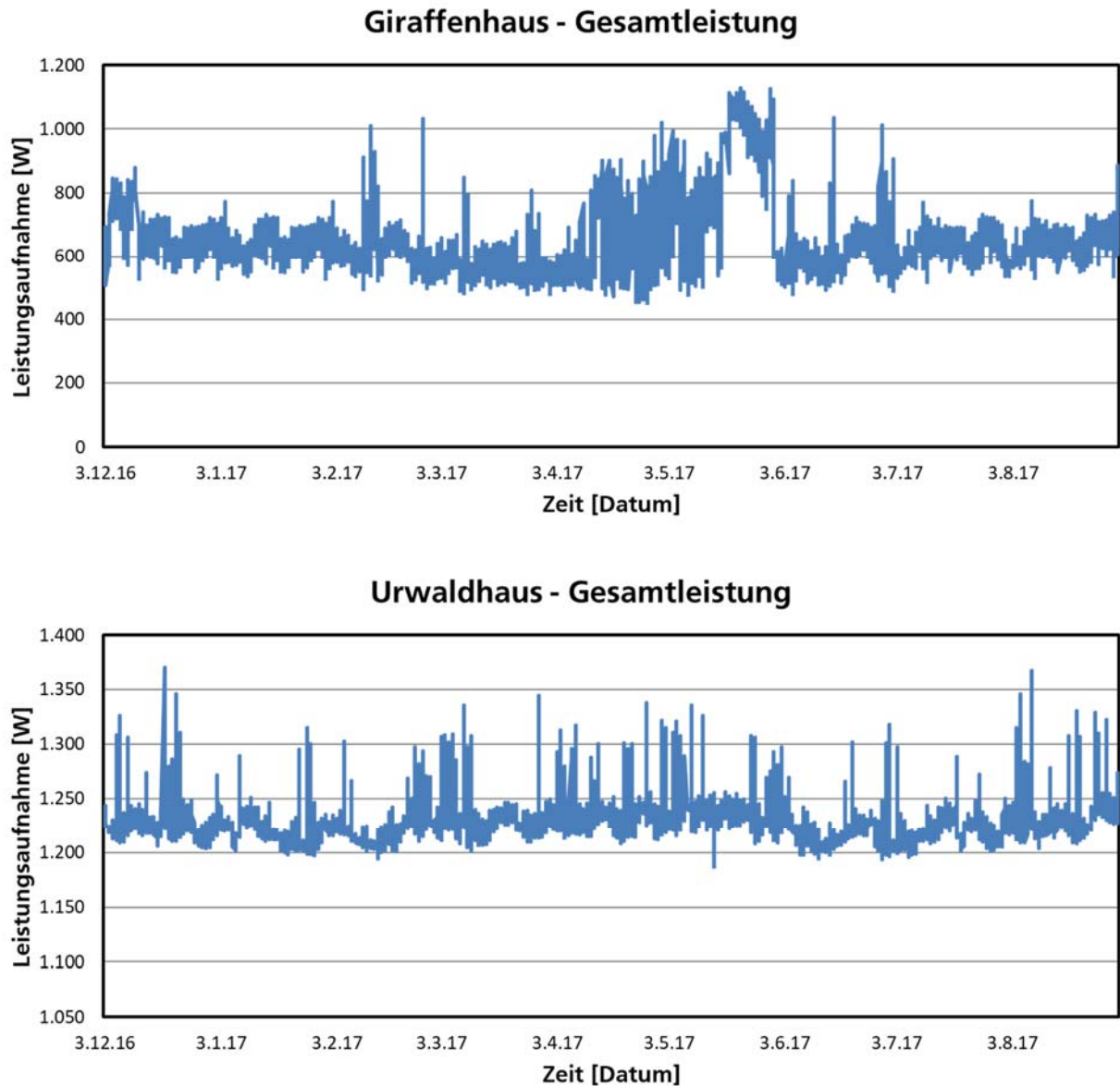
Bild 48: Vergleich gesamte Leistungsaufnahmen des Giraffenhaus (oben) und Urwald- hauses (unten).
