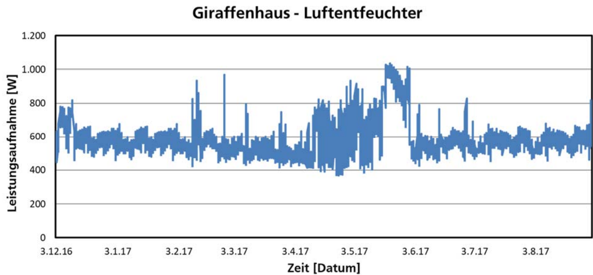
Bild 45: Giraffenhaushaus: Vergleich Leistungsaufnahme Luftversorgung - Luftentfeuchter.
