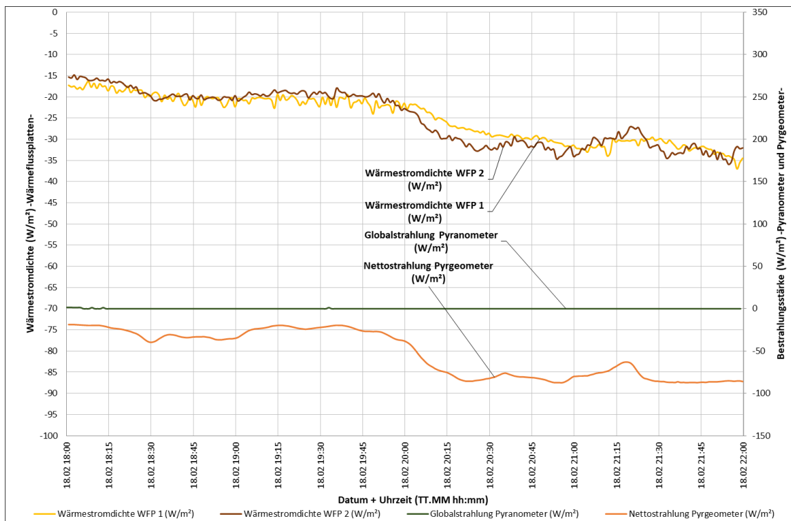
Abbildung 6.7: Auswertung 2.1.3.1 18.02. 18:00-22:00, Verlauf der Wärmestromdichten [11]
