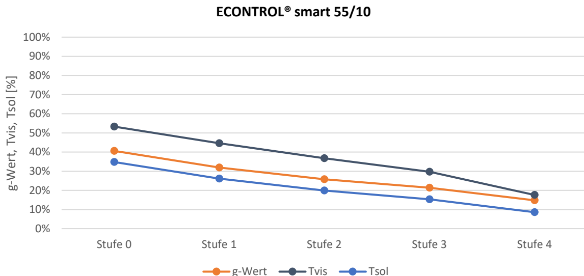
Abbildung 8.3: g-Wert, Tvis und Tsol der ECONTROL®-Verglasung in Abhängigkeit von der Schaltstufe (Quelle für CEN-Werte: EControl-Glas [28], NFRC-Werte basieren auf den Spektraldaten der EControl-Glas GmbH & Co. KG), Mittelwerte wurden berechnet mit den Programmen LBNL-Optics 5.1 sowie Window 7.4.6). Abbildung aus [29] entnommen.
