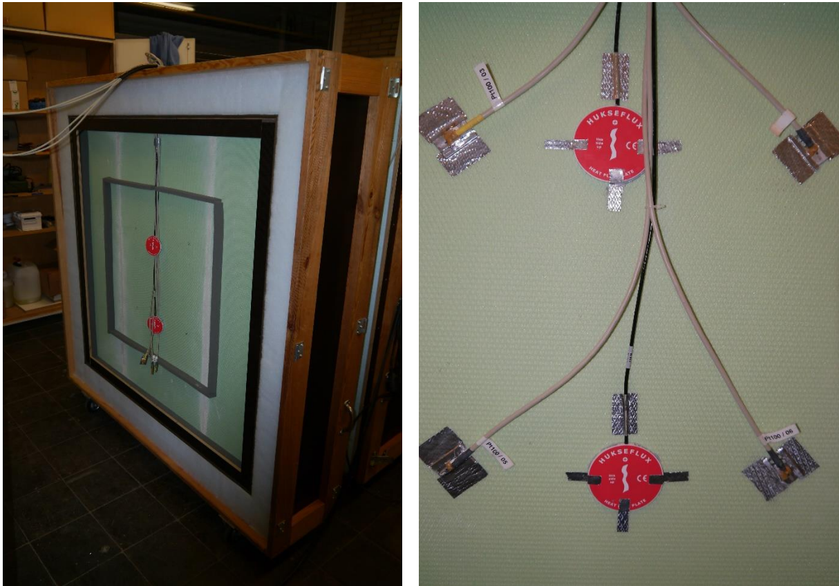
Abbildung 4.8: Warmseite der Hotbox mit eingebautem Referenzprobekörper (linkes Bild), auf dem anschließend die Sensoren befestigt wurden (rechtes Bild)
