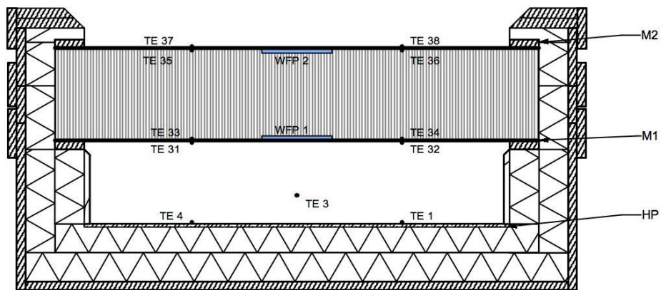
Abbildung 6.11: Schnitt durch den Dachprüfstand mit einem zweilagigen Aufbau mit Funktionsmaterial [11]
