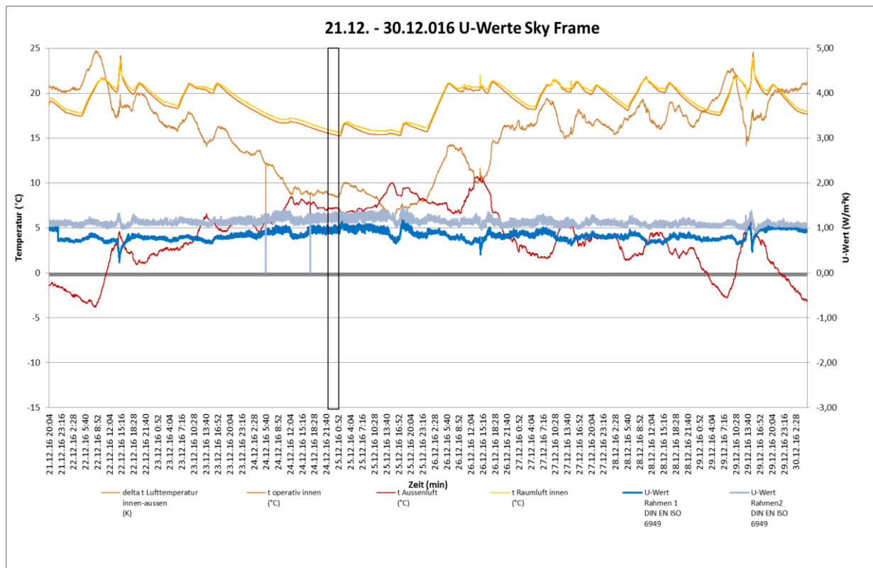
Abbildung 7.6: U-Werte Sky-Frame 21.12.-30.12.2016
