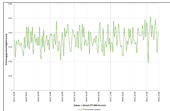
Abbildung 4.26: Strömungsgeschwindigkeit, bewölkter Tag, 25 % Heizleistung
