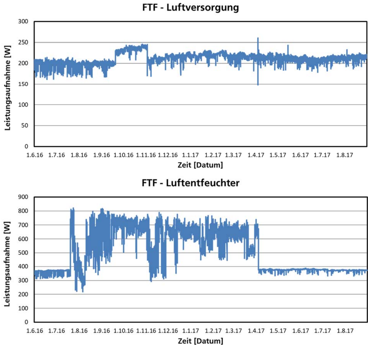
Bild 43: FTF: Vergleich Leistungsaufnahme Luftversorgung - Luftentfeuchter.
