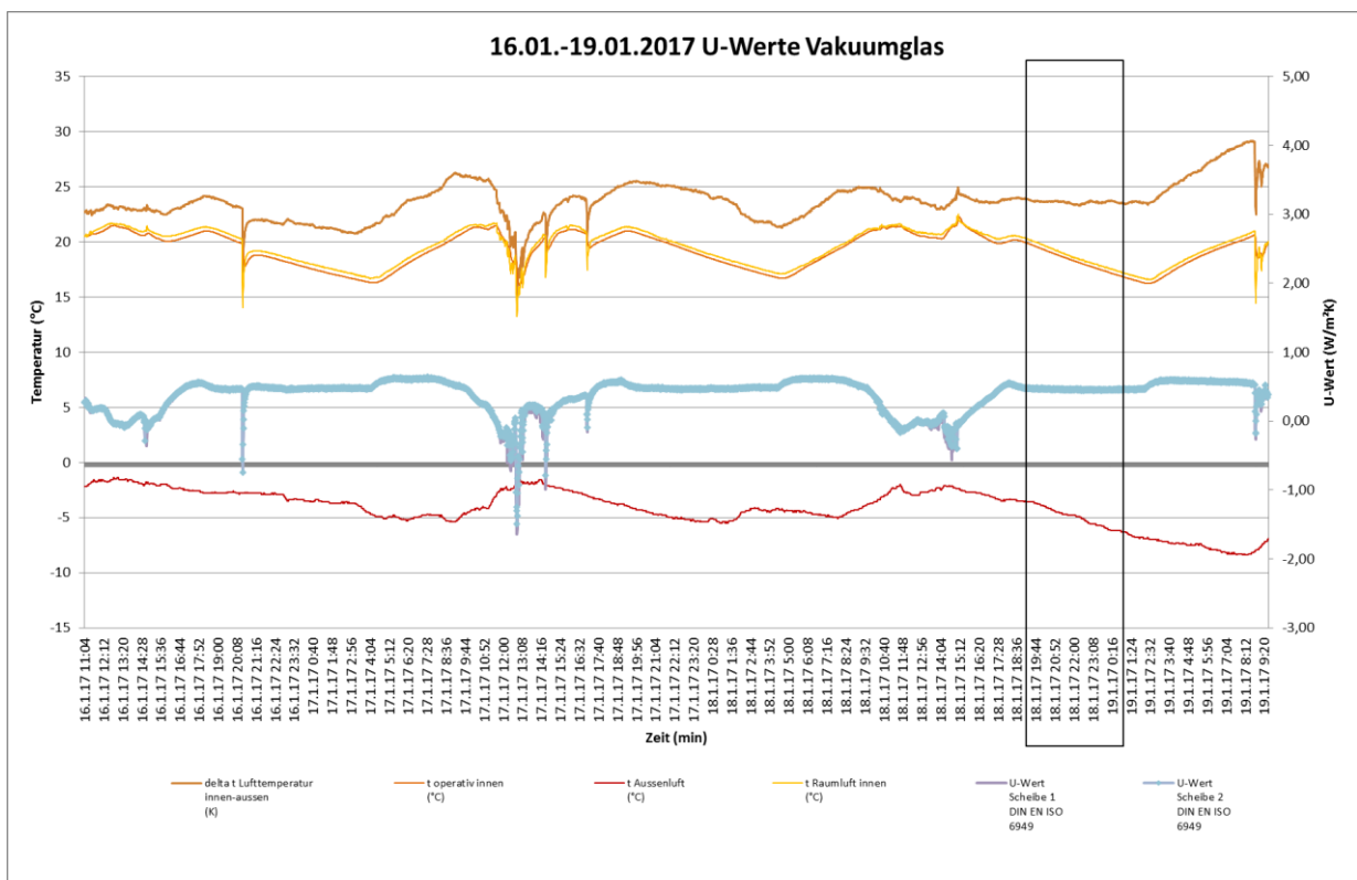
Abbildung 7.17: U-Werte Vakuumglas 16.1.-19.1.2017
