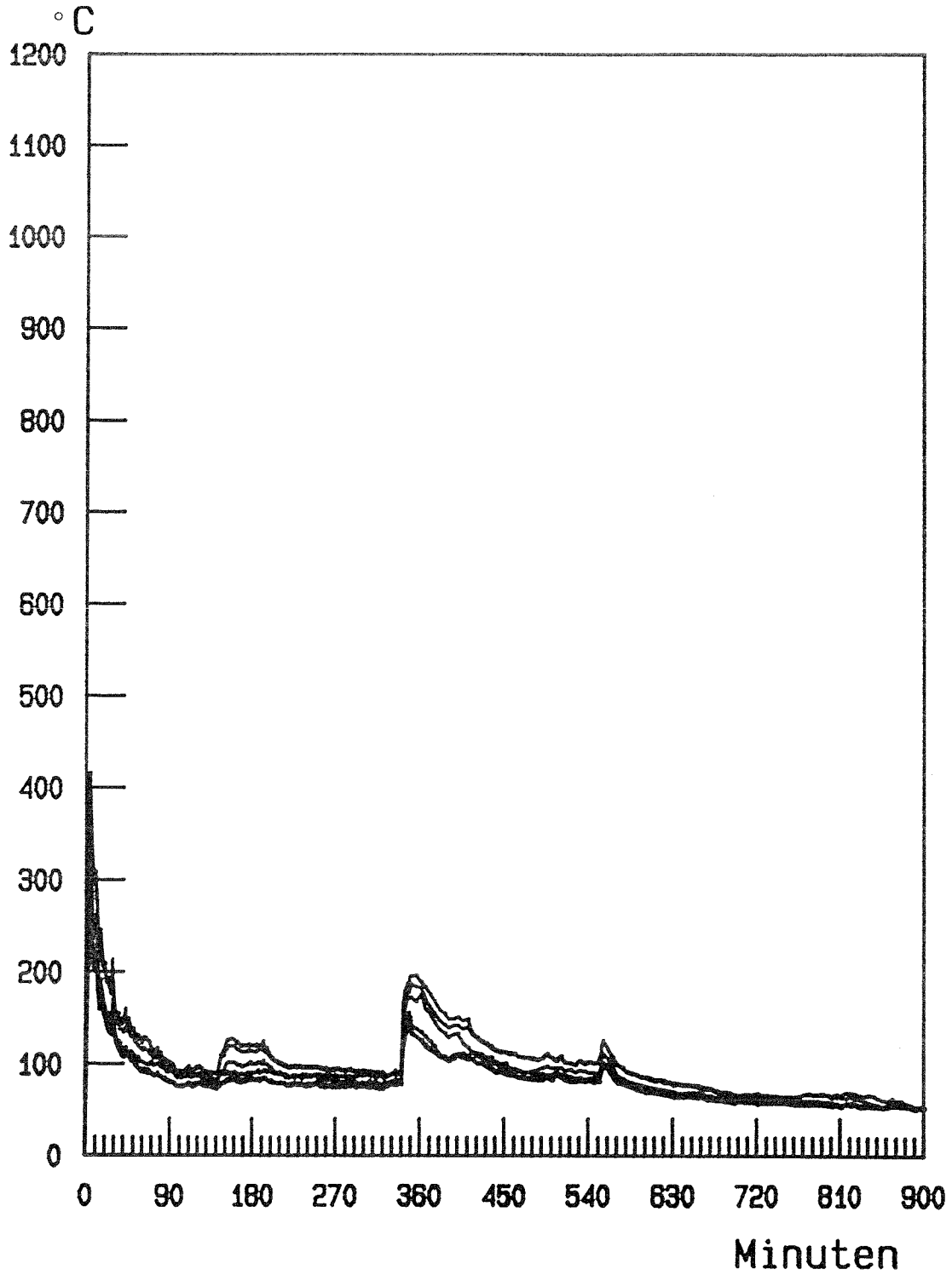
Temperaturverlauf in der Thermosäule "D" (Mess-Stellen 7 bis 13)
