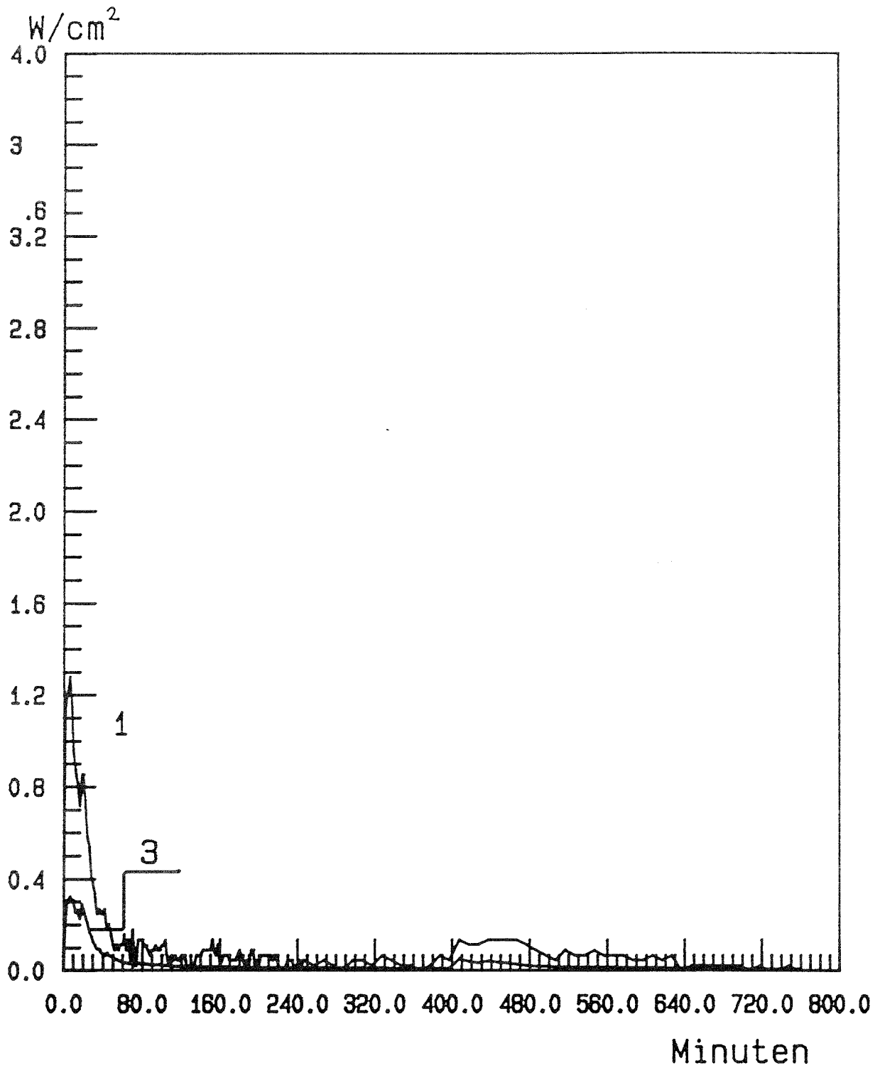
Wärmestromdichten unter der Decke und im Bereich des Brandraumverschlusses
