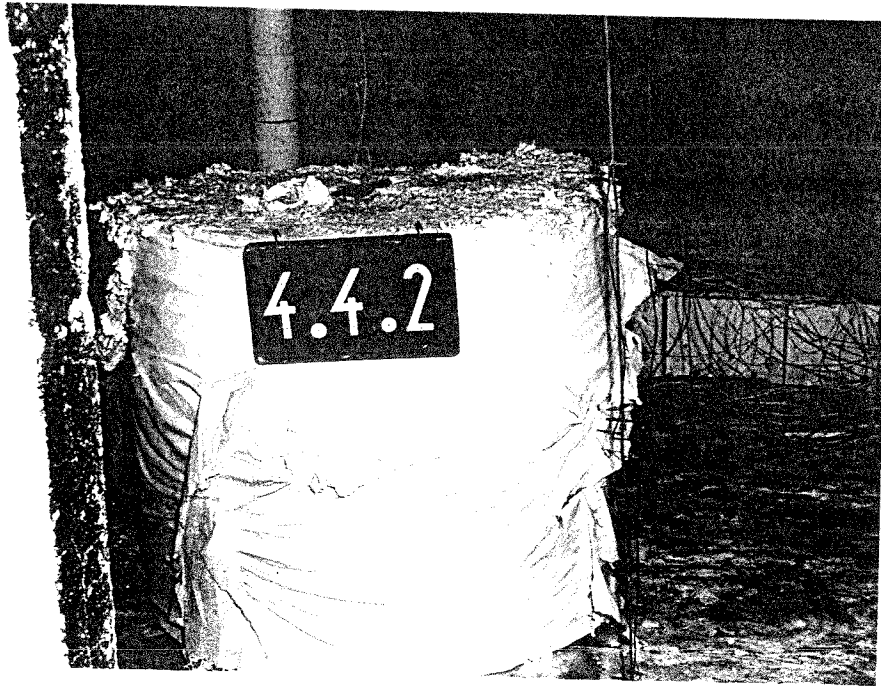
Abb. 1: Sicht in den Brandraum vor dem Versuch
